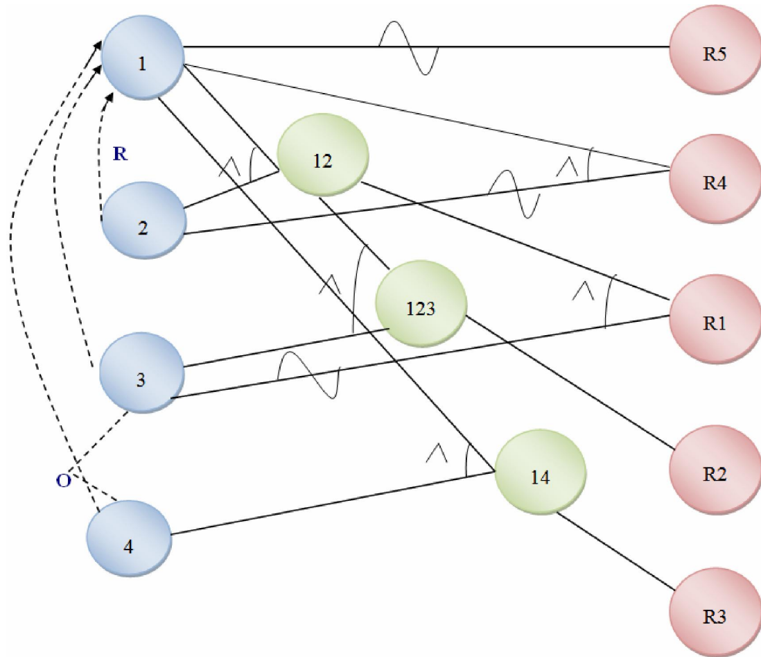
Hình 3.1 Đồ thị nguyên nhân – kết quả:
