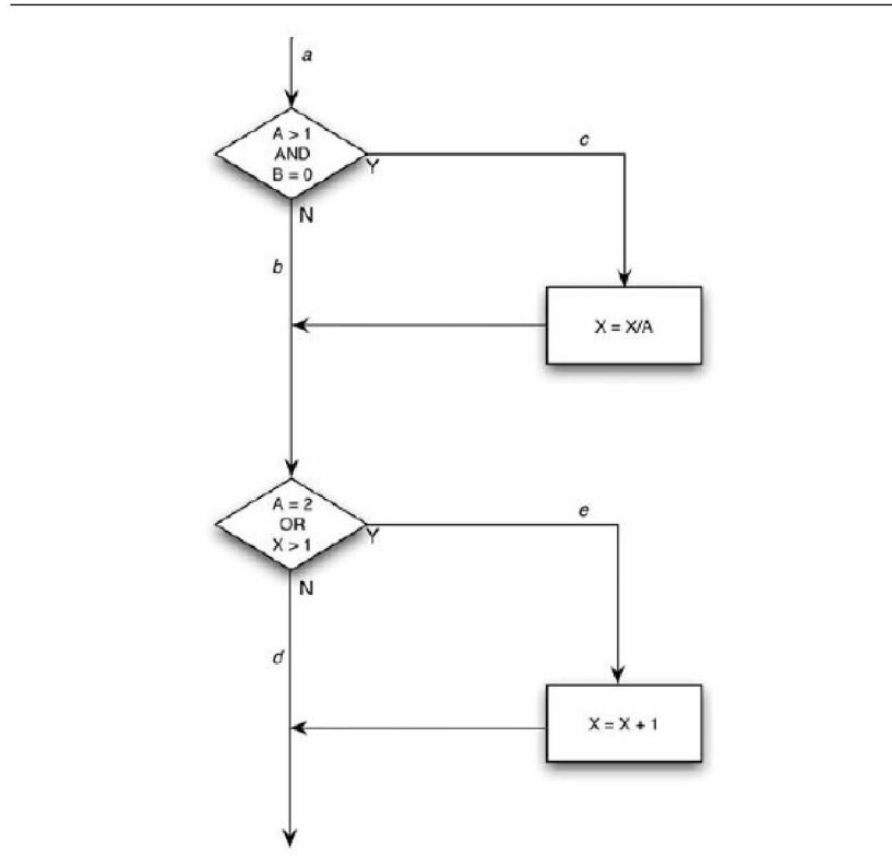
Hình 2.1 Một chương trình nhỏ để kiểm thử
