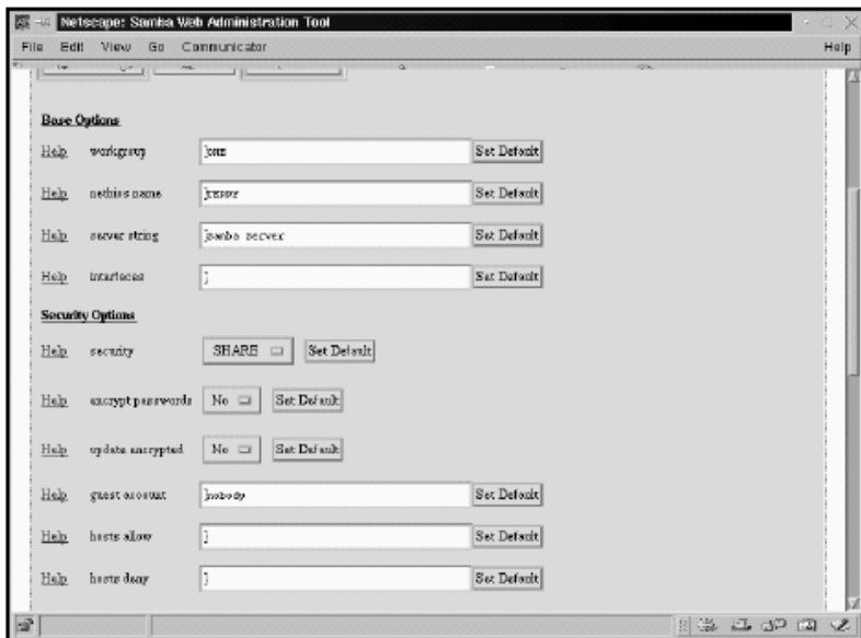
Base và Security Options
