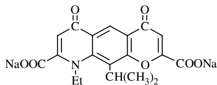
Nedocromilnatri
