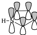
Cấu tạo của pyrrol
