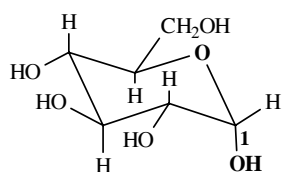
Dạng C1 \alpha -D-Glucopyranose
