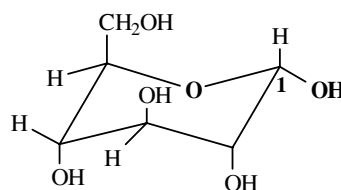
Dạng 1C \alpha -D-Glucopyranose
