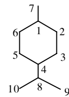
Khung p-Mentan
