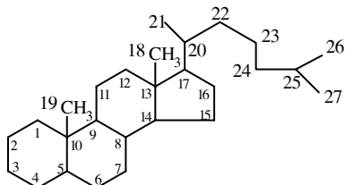
Đánh số trên khung Cholestan
