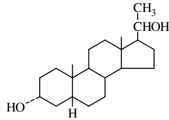
Pregnan-3 alpha:20 alpha -diol (5β -Pregnan-3 α :20α -diol)
