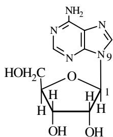
Adenosin ( Ribose + Adenin )
