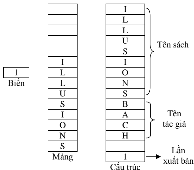
Hình 19.1. Sự khác nhau giữa một biến, một mảng và một cấu trúc.
