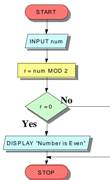
Hình 1.7 : Kiểm tra số chẵn
