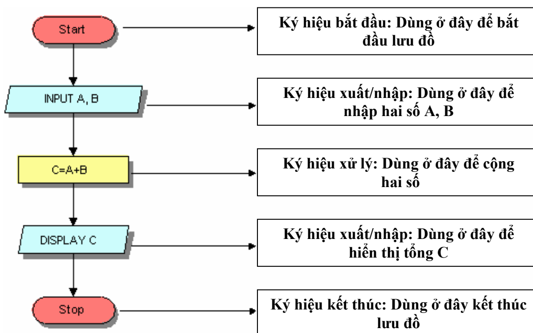
Hình 1.5: Lưu đồ cộng hai số
