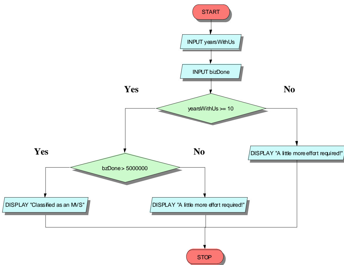
Hình 1.9: Câu lệnh IF lồng nhau
