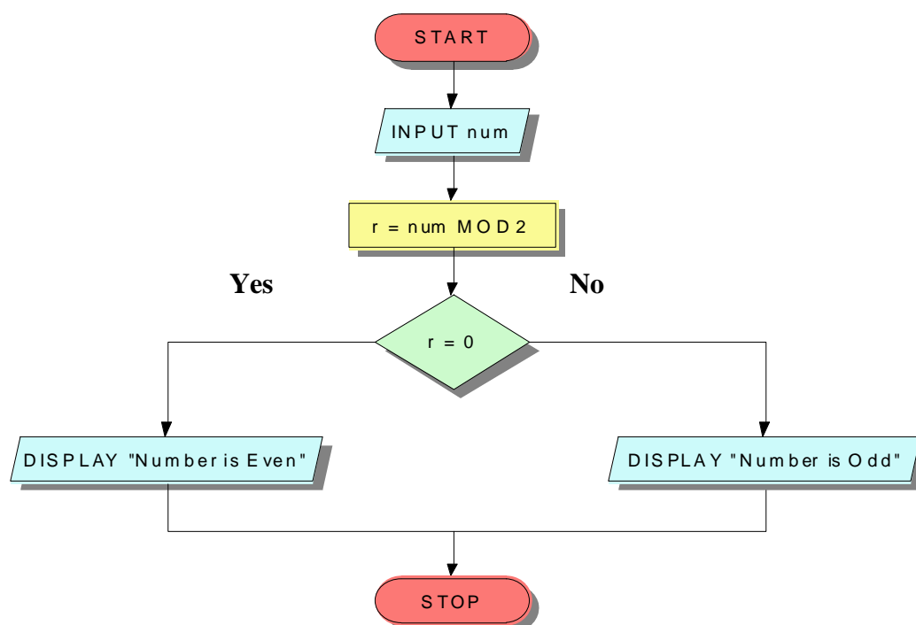
Hình 1.8: Số chẵn hay số lẻ
