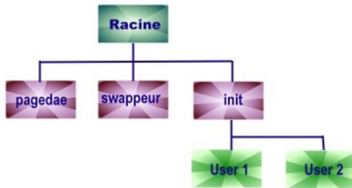
Hình 2.5 Một cây tiến trình trong hệ thống UNIX
