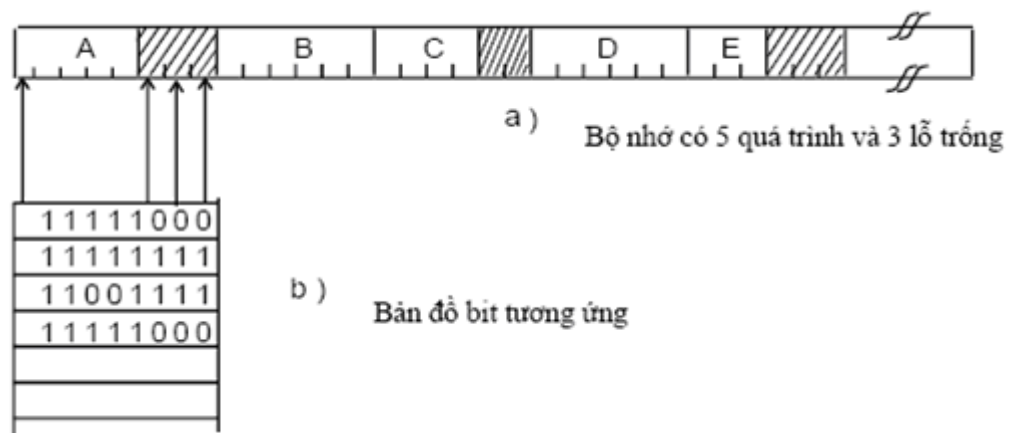
1 Hình 3.6 Quản lý bộ nhớ bằng bản đồ bit
