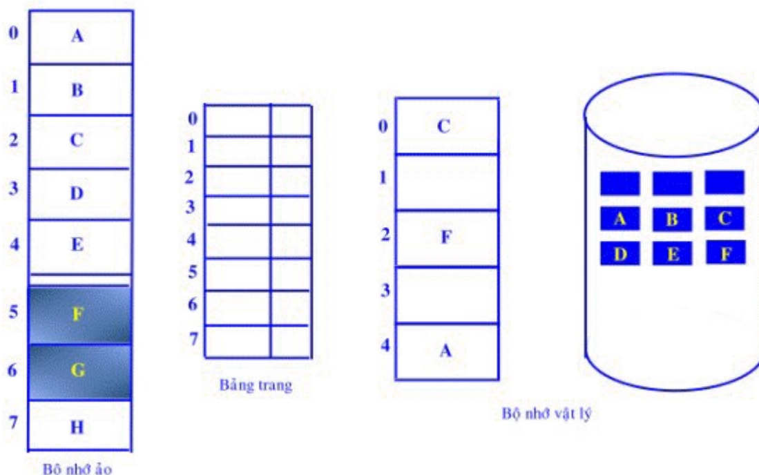
Hình 3.26 Bảng trang với một số trang trên bộ nhớ phụ
