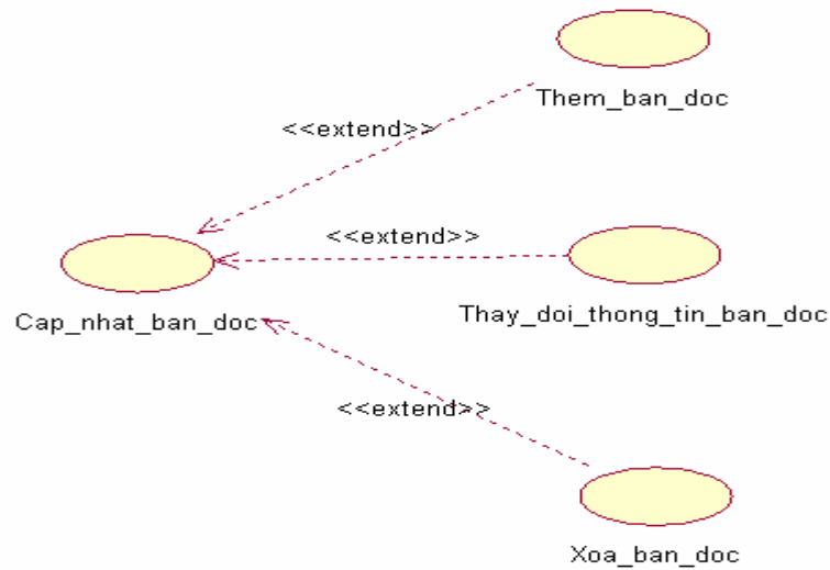
Hình 3.3: Phân rã use case Cập nhật bạn đọc
