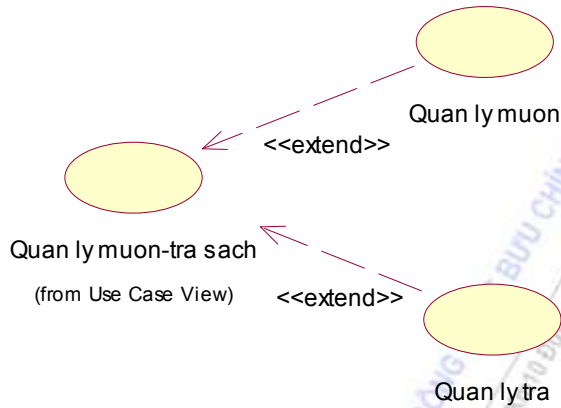
Hình P.3: Phân rã use case Quản lý mượn trả sách
