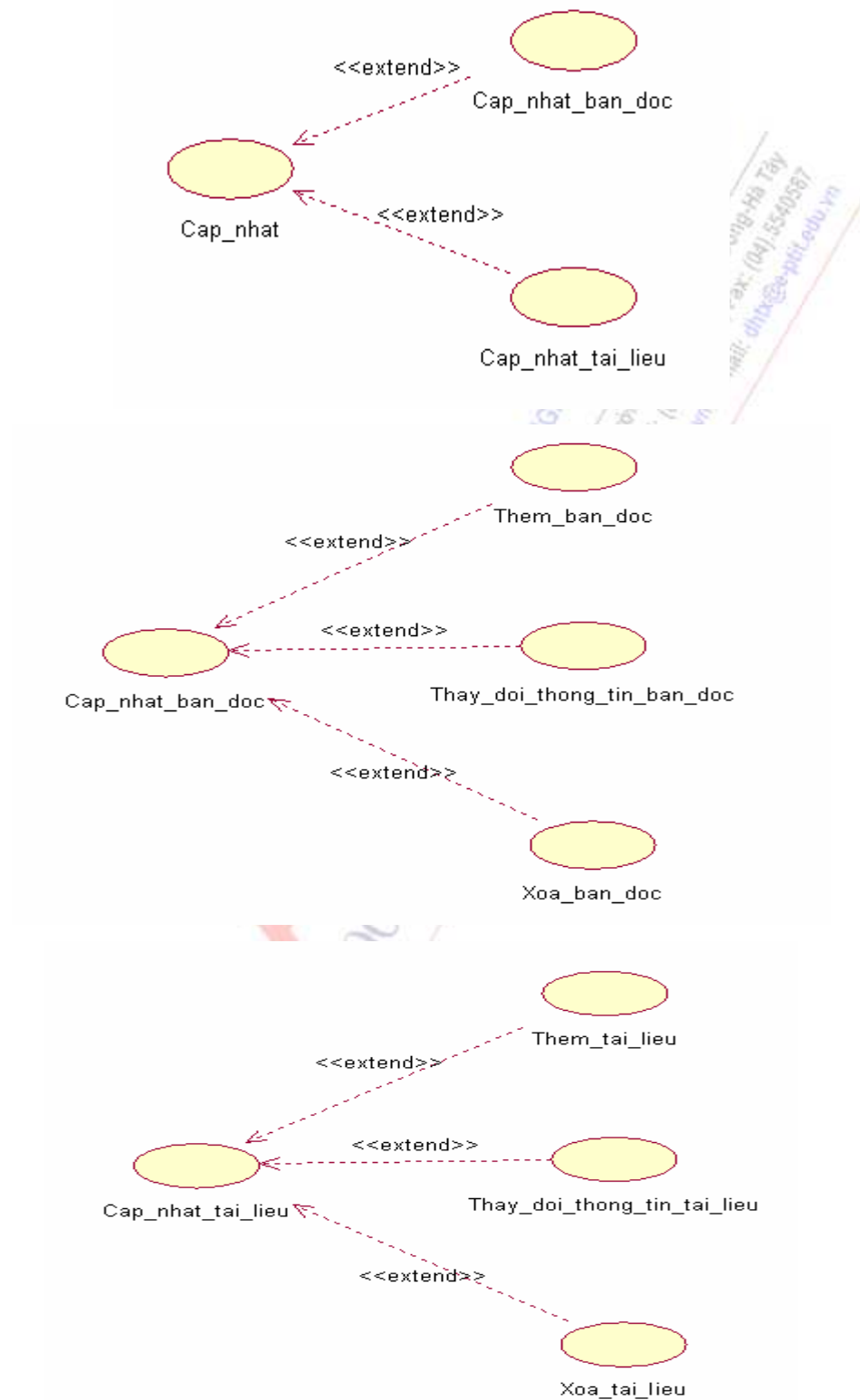
Hình P.2: Phân rã use case cập nhật
