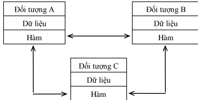
Hình 3-3. Tổ chức dữ liệu và hàm trong chương trình HĐT
