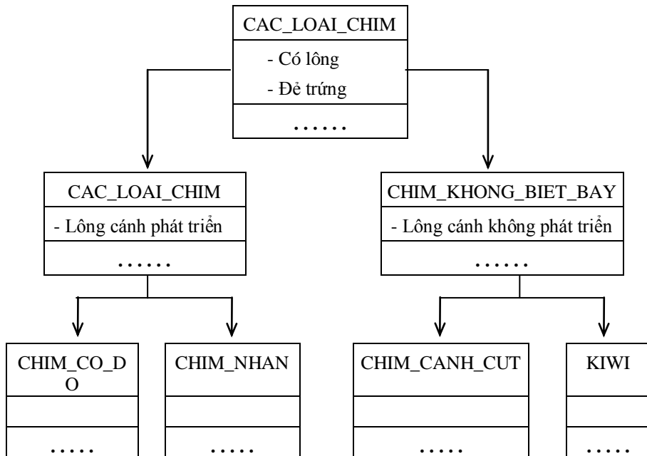
Hình 2-1. Quan hệ kế thừa
