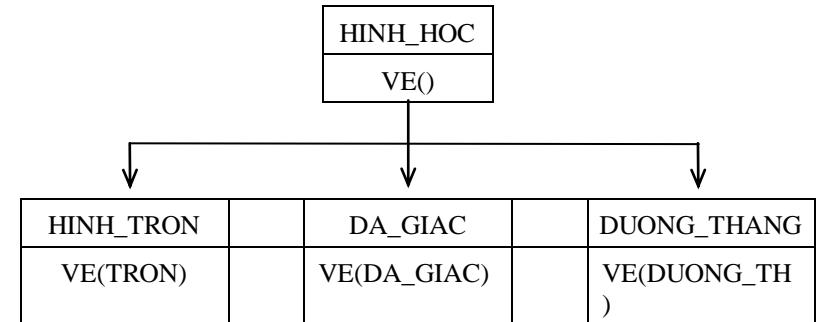
Hình 3-5. Tương ứng bội của hàm VE()
