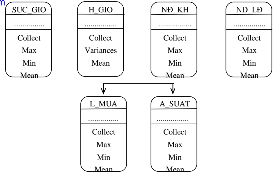
Hình 2-7. Mô tả quan hệ của các lớp đối tượng "mềm"
