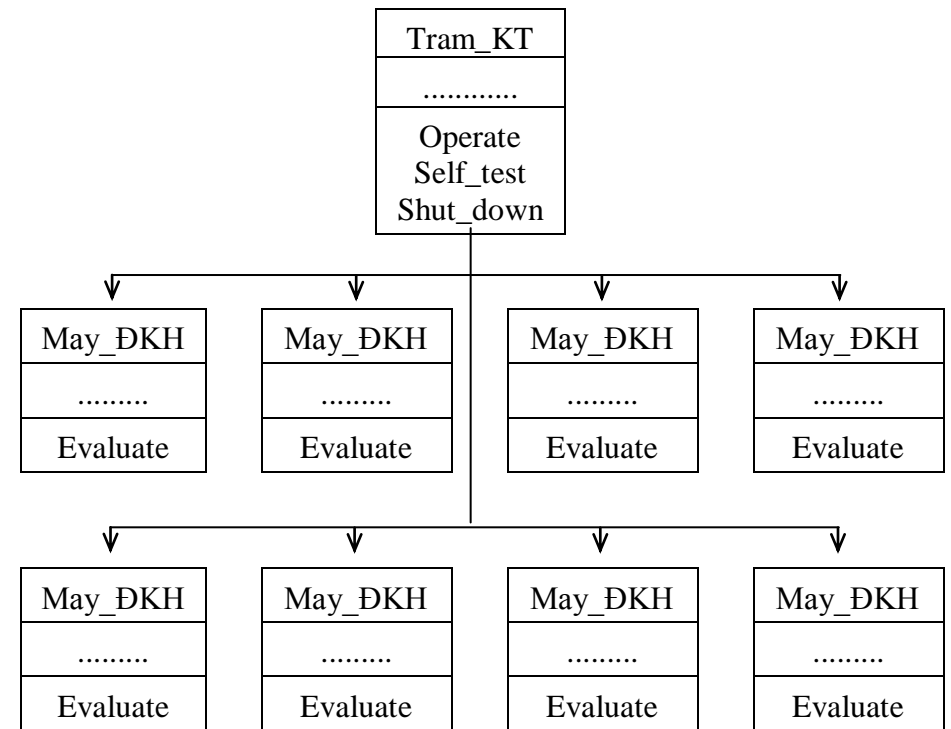
Hình 2-6. Cấu trúc phân cấp của phần cứng
