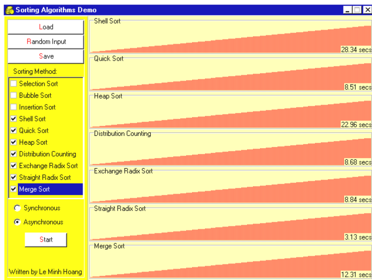
Hình 16: Cài đặt các thuật toán sắp xếp với dữ liệu lớn, cho phép chạy các thuật toán theo kiểu song song (Synchronous) hoặc tuần tự (Asynchronous), Straight Radix Sort tỏ ra nhanh nhất
