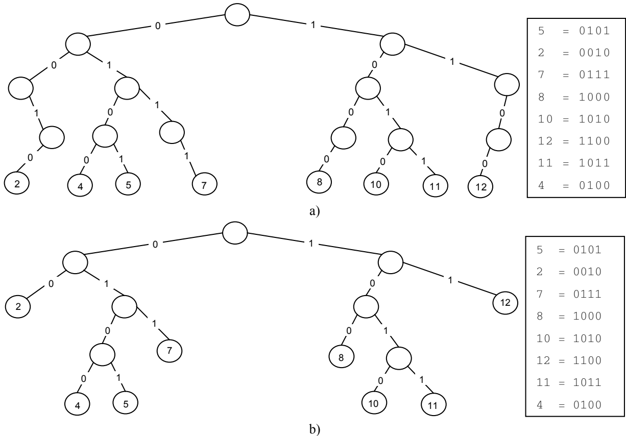
Hình 22: Cây tìm kiếm cơ số a) và Trie tìm kiếm cơ số b)
