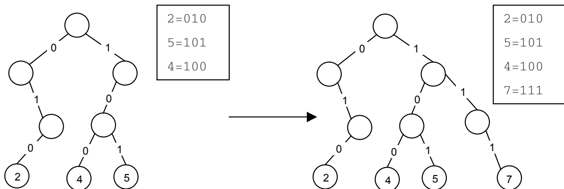
Hình 20: Với độ dài dãy bit z = 3, cây tìm kiếm cơ số gồm các khoá 2, 4, 5 và sau khi thêm giá trị 7
