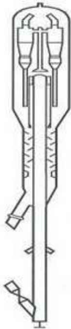
Hình H-1.22. Bộ phận trộn sơ bộ và phân tán xúc tác
