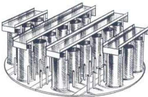
H-5.27E. Hệ thống phân phối dạng ống chảy tràn
