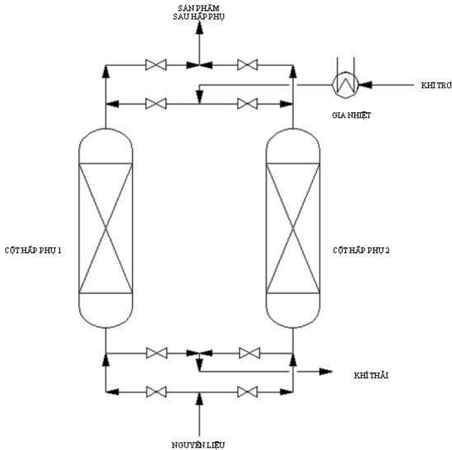
Hình H-6-5-Sơ đồ nguyên lý chu trình hấp phụ sử dụng khí trợ nhả hấp phụ
