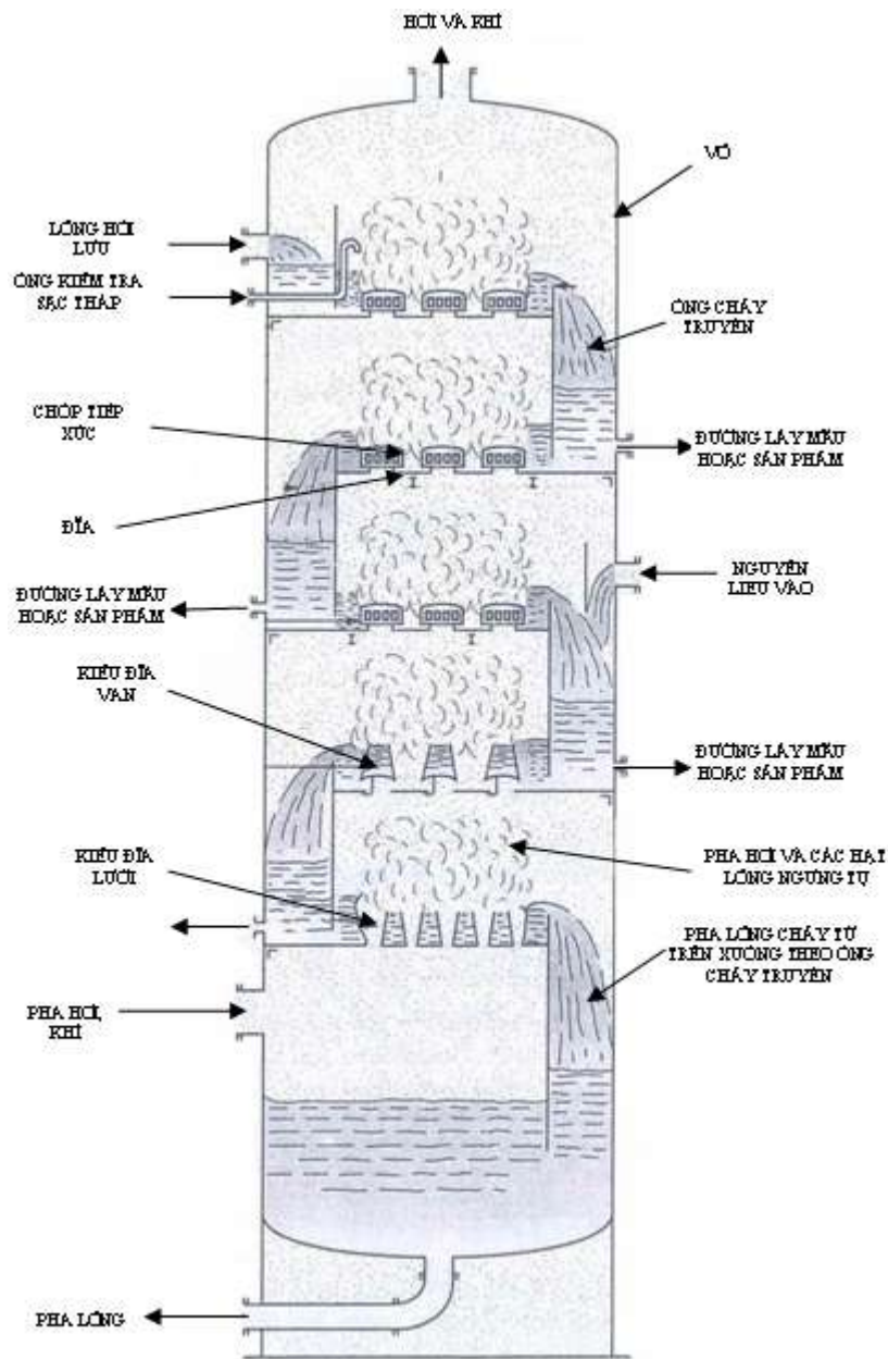
Hình H-5.7- Cấu tạo chung tháp chưng cất dạng đĩa (mặt cắt ngang)
