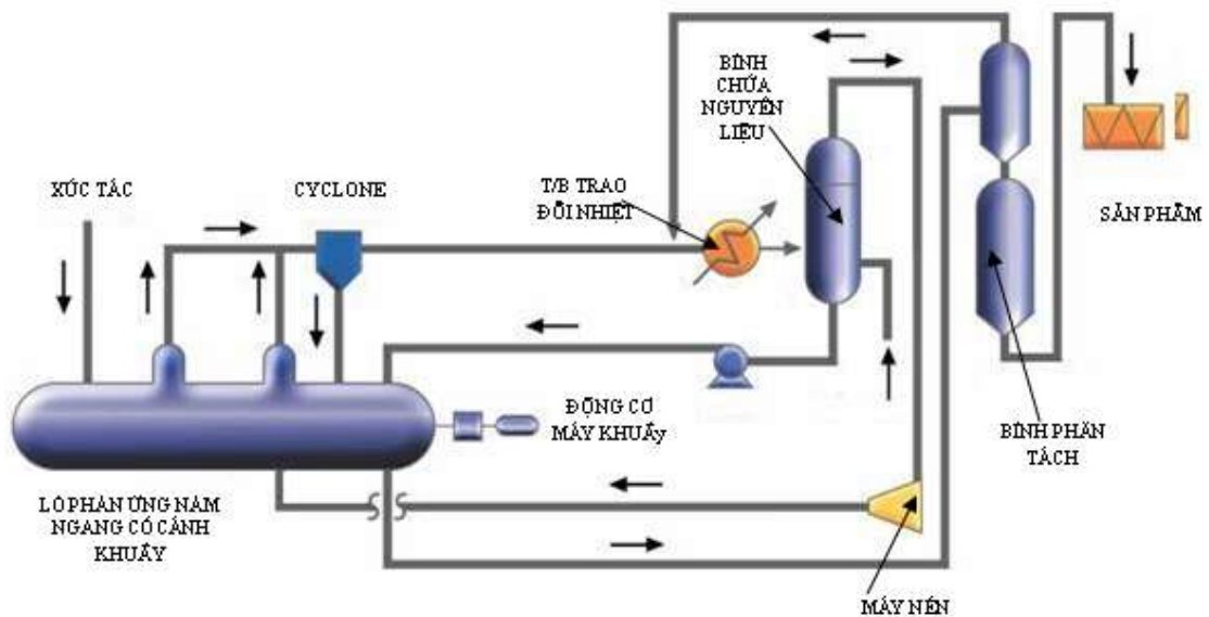
Hình H-1.54 Thiết bị phản ứng khuấy trộn kiểu nằm ngang
