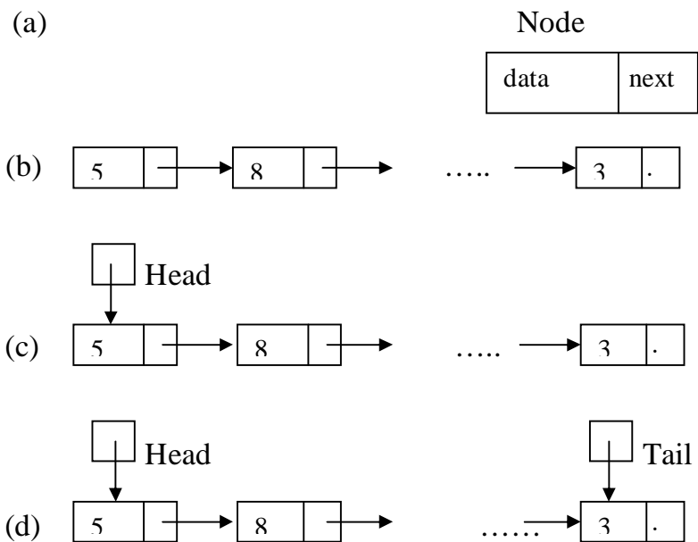
Hình 5.3. a) Một thành phần của DSLK. b) DSLK chứa các số nguyên. c) DSLK với một con trỏ ngoài Head d) DSLK với hai con trỏ ngoài Head và Tail.
