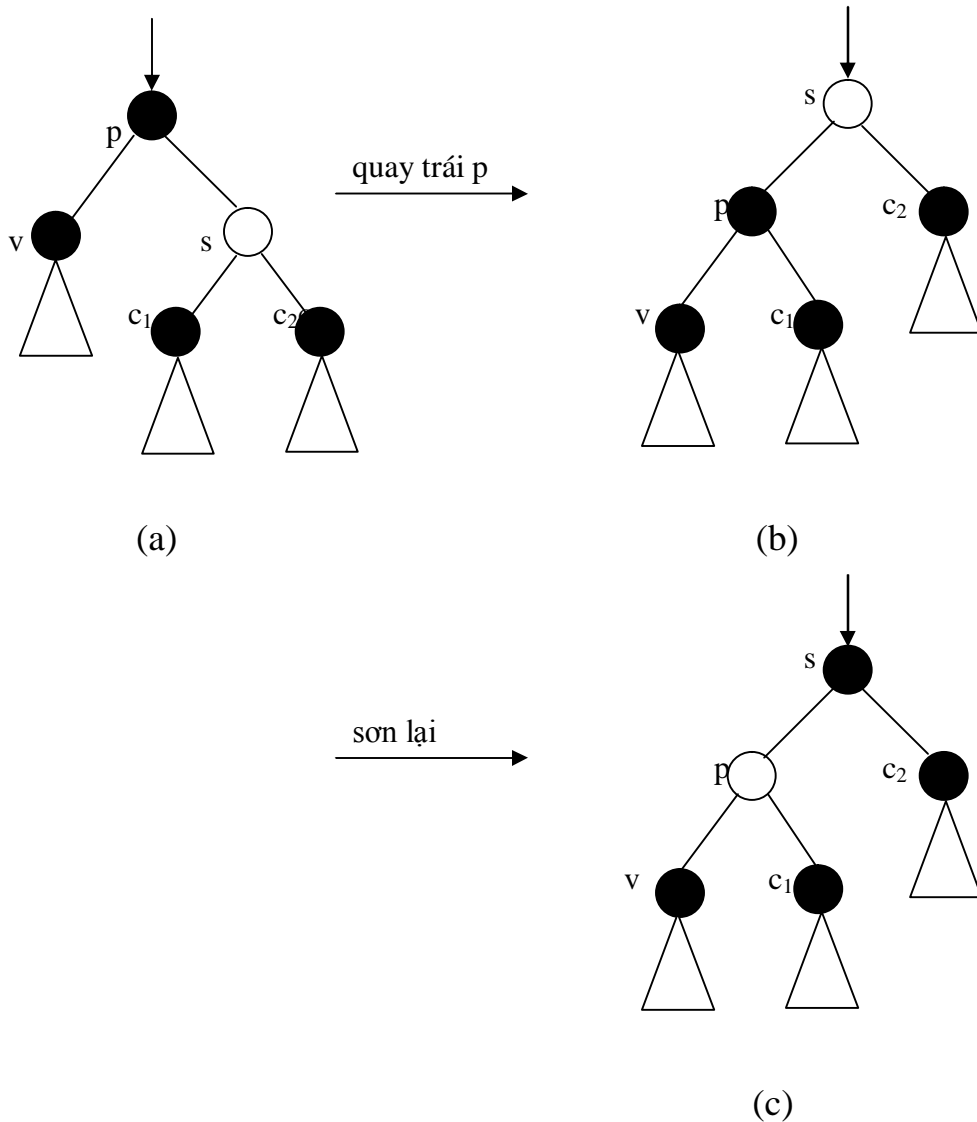
Hình 11.13. Mẫu điều chỉnh 4.
