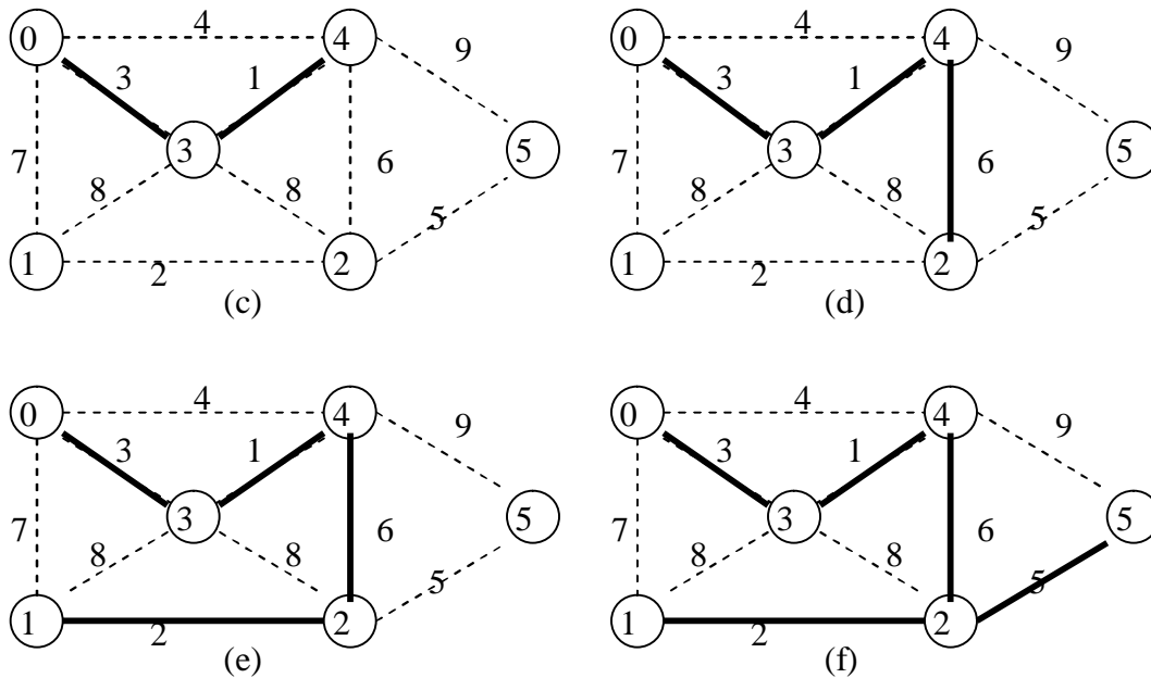
Hình 18.9. Phát triển cây T theo thuật toán Prim.
