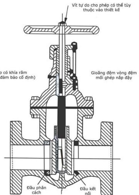
Van chặn hai đĩa ty cố định
