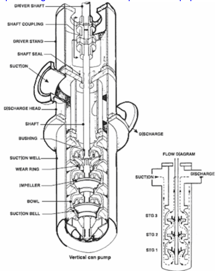
Bơm đa cấp trực đứng
