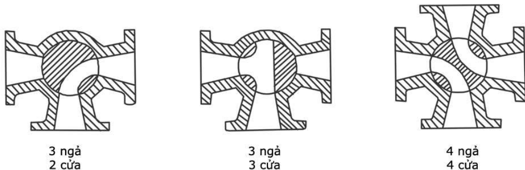
Các kiểu van nhiều cửa
