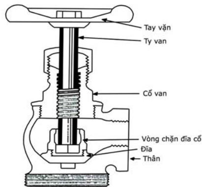
Van cầu góc với mép bắt bulông
