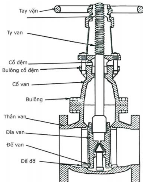
Van chặn có bích hai đĩa ty van đi lên áp suất 150 psig
