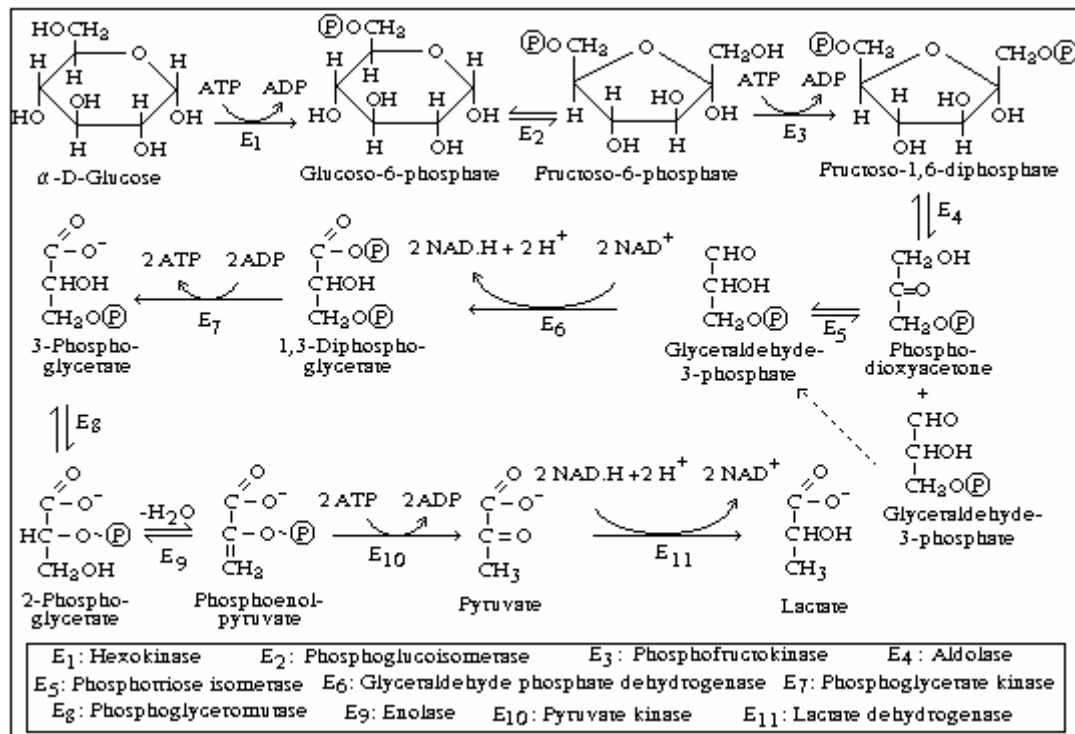
Hình IX.4: Sơ đồ tổng quát của quá trình glycolys
