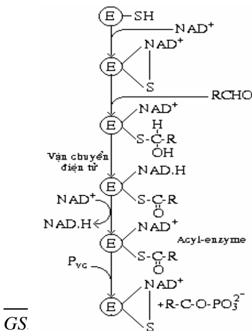
Hình IX.5. Cơ chế tác dụng của glyceraldehyde phosphate
