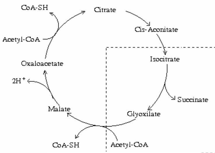
H10.5. Chu trình glyoxylate
