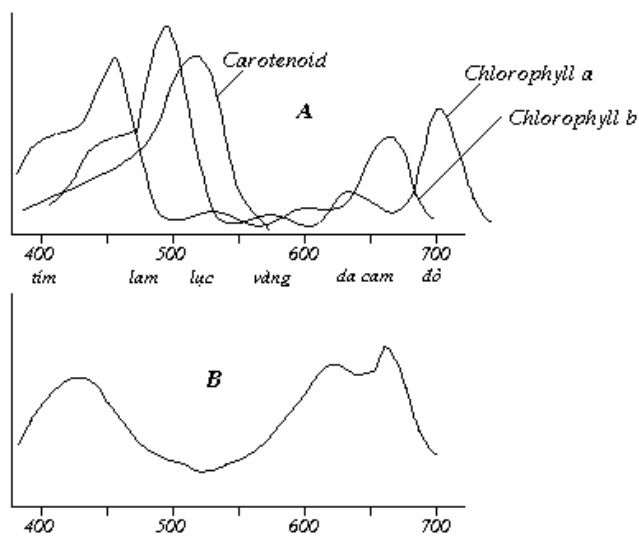
HÌNH IX.12. QUANG PHỔ HẤP THỤ (A) VÀ QUANG PHỔ HOẠT ĐỘNG (B) CỦA CHLOROPHYLL
