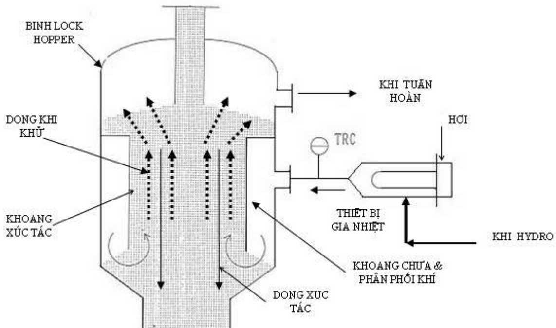
Hình H-1.45 Cấu tạo nguyên lý hoạt động vùng khử xúc tác
