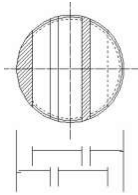
C-kiểu ba dòng chảy trên đĩa
