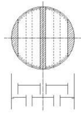
Dkiểu bốn dòng chảy trên đĩa
