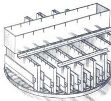
H-5.27F. Hệ thống phân phối dạng máng Hình răng cưa
