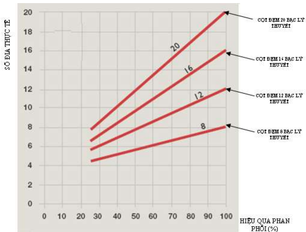
Hình H-5.26. Ảnh hưởng của phân phối chất lỏng đến hoạt động tháp đệm
