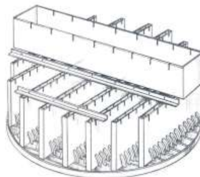
H-5.27D. Hệ thống phân phối dạng máng có đầu ống phân phối
