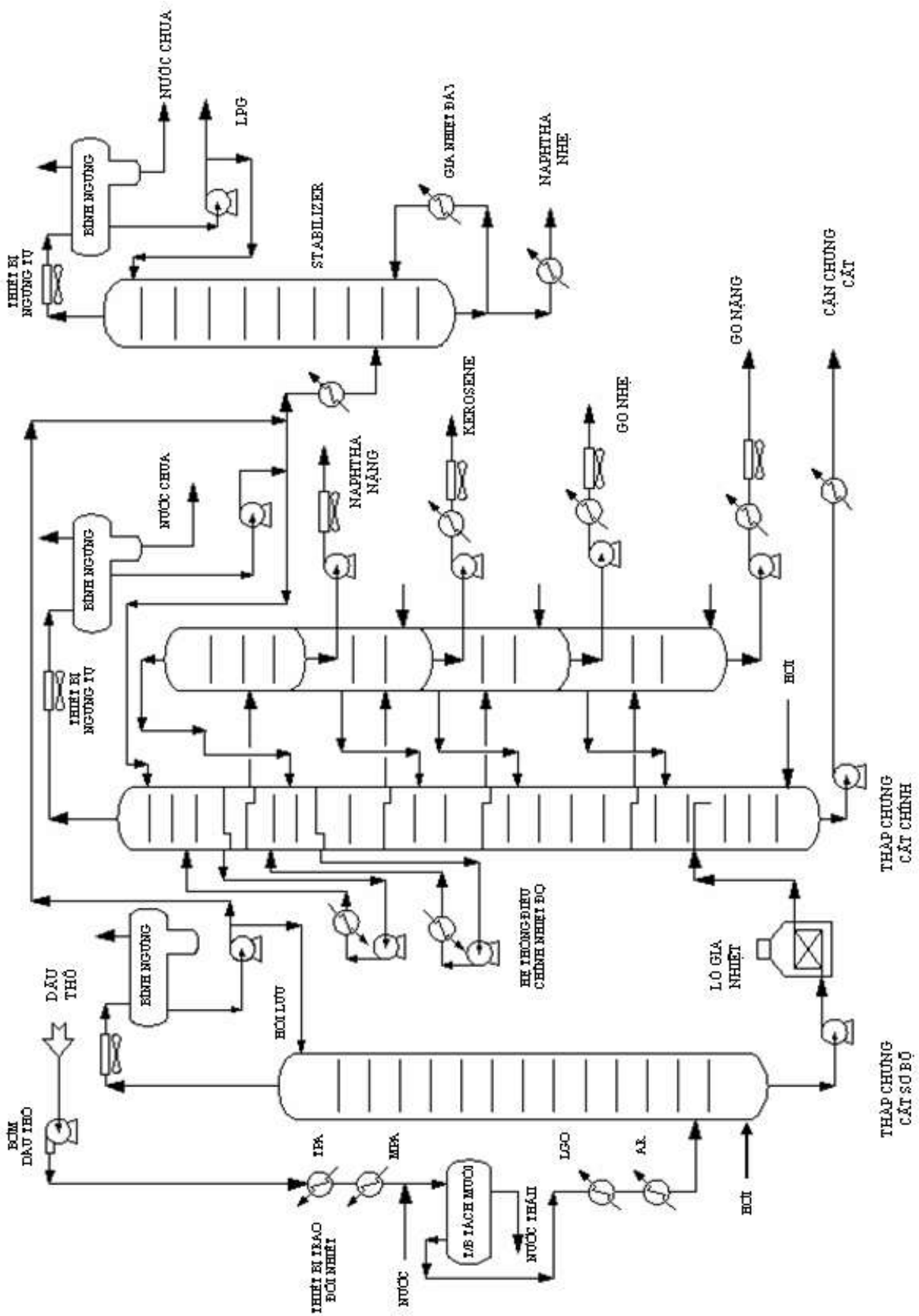
Hình H-5.30. Sơ đồ công nghệ phân xưởng chưng cất dầu thô ở áp suất khí quyển với một tháp chưng cất chính
