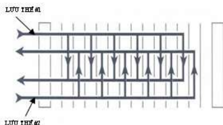
Hình H-2.16A Sơ đồ bố trí dòng chảy trong thiết bị (dòng chảy đơn)
