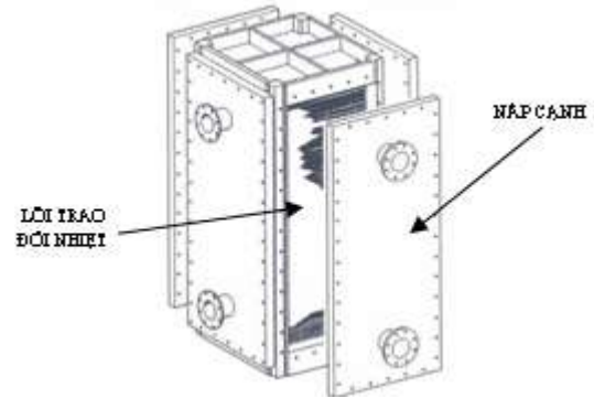
Hình H-2.21B-Cấu tạo khung (các nắp cạnh và cửa dẫn lưu thể vào/ ra)
