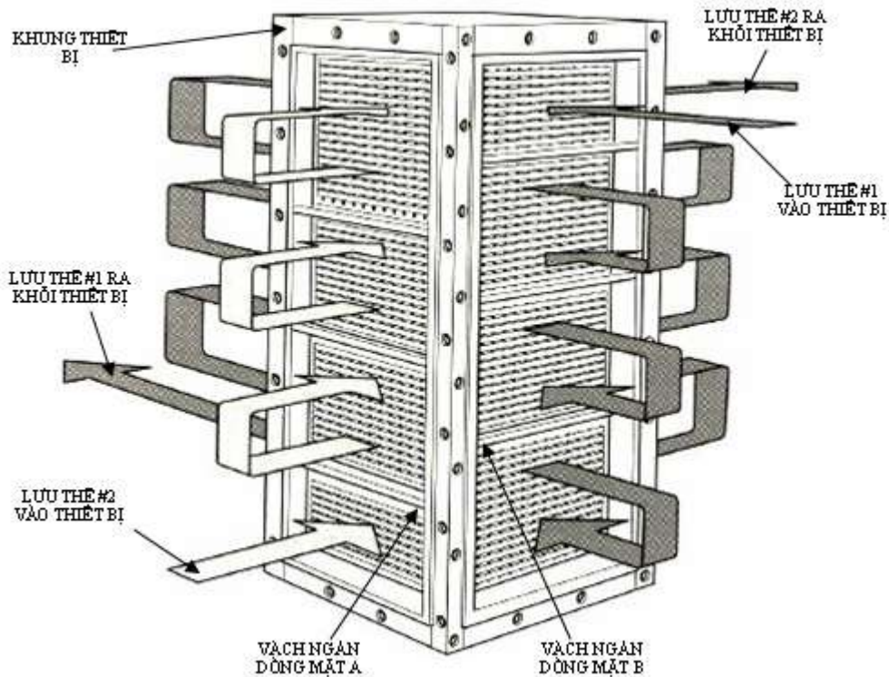
Hình h-2.22. Sơ đồ nguyên lý hoạt động và bố trí dòng trong thiết bị trao đổi nhiệt tấm bản hàn kín
