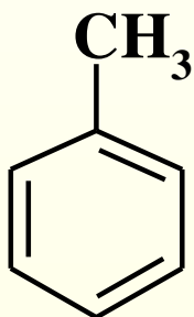
metylbenzen (toluen)
