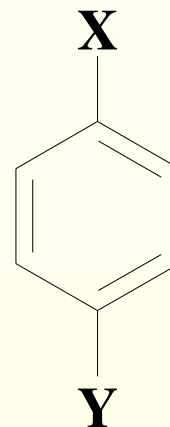
para
