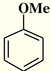
metoxybenzen (anisol)
