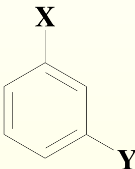
meta
