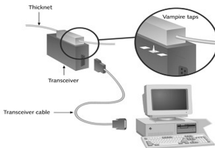
Hình 3.5 Sơ đồ mạng dùng cáp đồng trục dày
