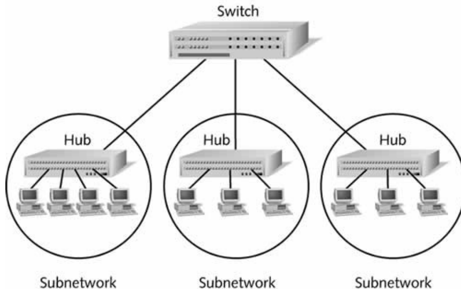
Hình 5.10 Mạng Ethernet chuyển mạch
