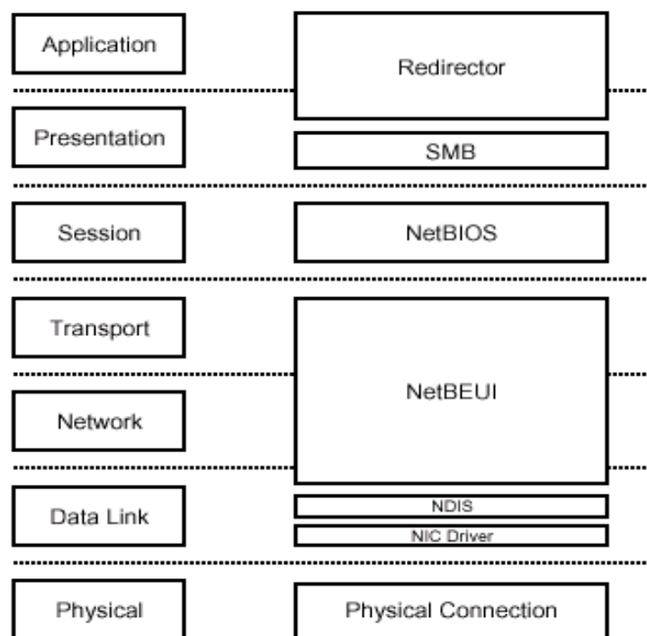
Hình 4.3 So sánh giao thức Microsoft Networking với mô hình OSI NetBIOS : Network Basic Input Output System
