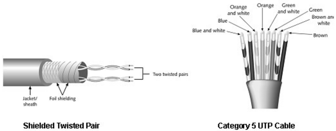
Hình 3.7 Cáp xoắn đôi
