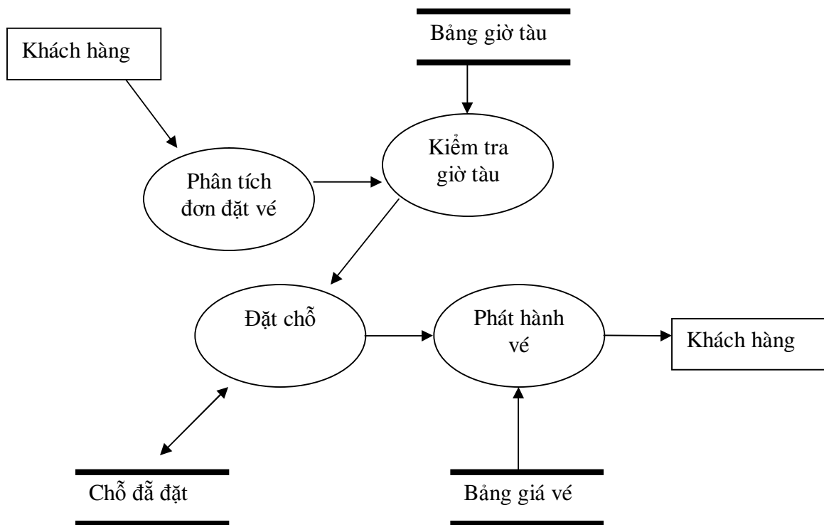
DFD mức 1
