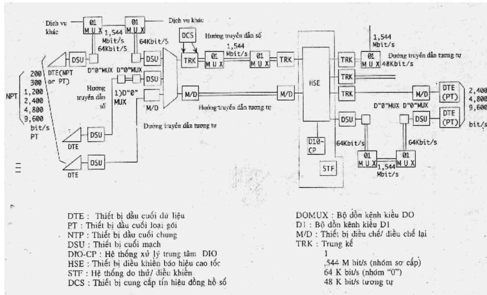
Hình 2.24. Phương pháp phục hồi mạng chuyển mạch gói
