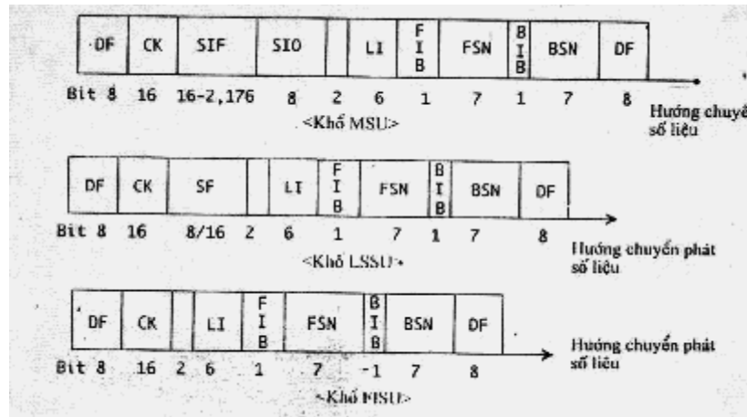
Hình 2.33. Kích thước của đơn vị tín hiệu SS No.7
