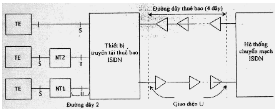
Hình 3.63. Thiết lập thiết bị truyền tải thuê bao của mạng
