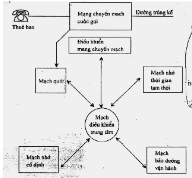
Hình 2.14. Thiết lập hệ thống tổng đài điện tử.
