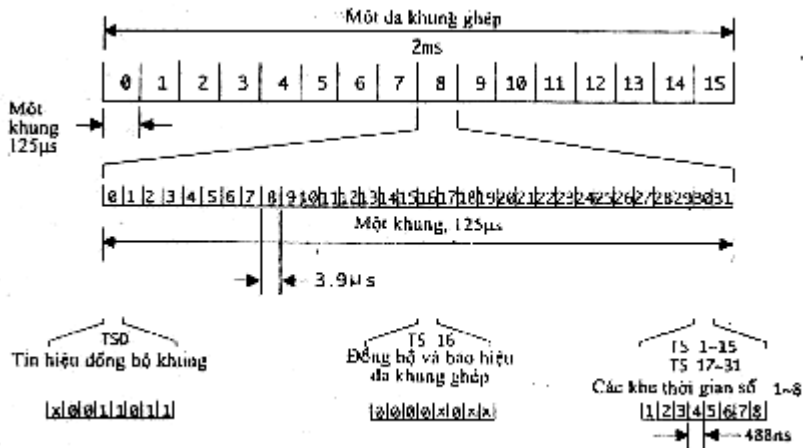
Hình 3.29. Cấu hình khung của nhóm sơ cấp theo kiểu E1
