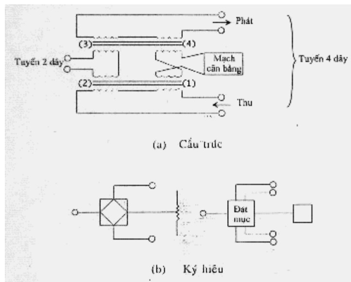
Hình 3.46. Cuộn dây hybrid
