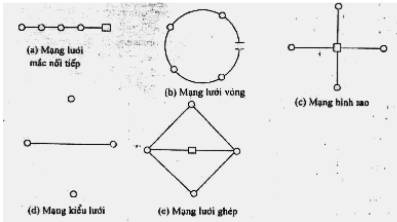
Hình 2.16. Các kiểu mạng lưới đường dây
