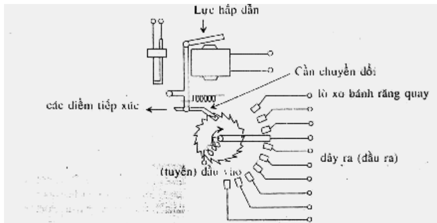
Hình 2.3 Nguyên lý một chuyển mạch xoay
