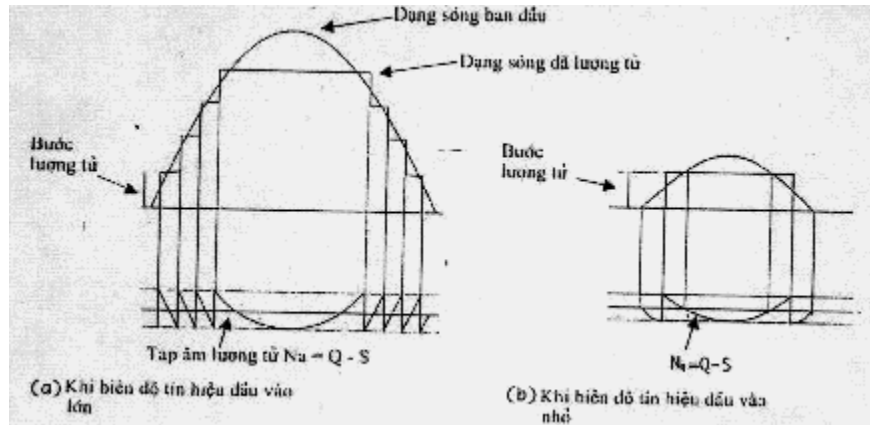
Hình 3.11. Tạp âm lượng tử theo biên độ tín hiệu đầu vào
