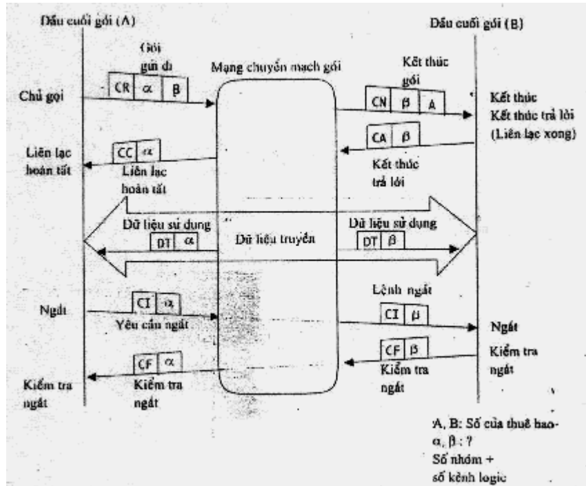
Hình 2.26. Thủ tục truyền tin gói
