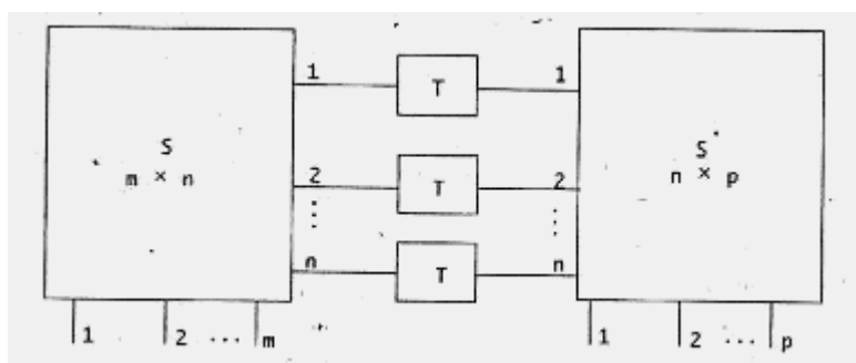
Hình 2.9. Cấu trúc mạng S-T-S.
