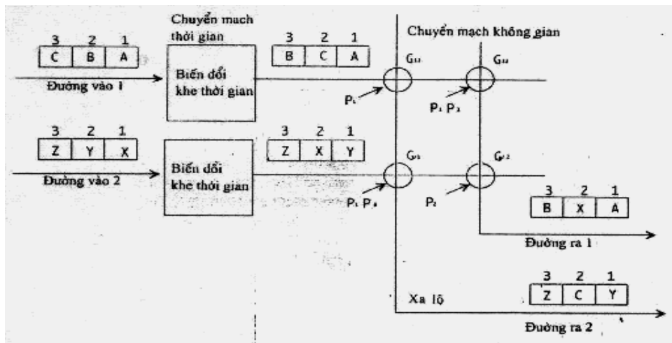
Hình 2.21. Nguyên tắc hệ thống chuyển mạch số phân chia thời gian
