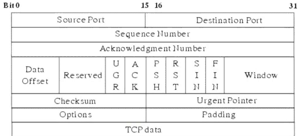
Hình 7.5: Dạng thức của segment TCP
