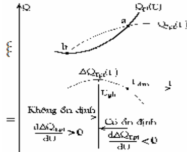
Hình 2 - Đặc tính Q U và ΔQ U
