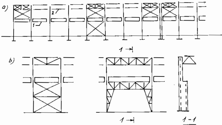
Hình 1.7. Bố trí giằng cột: a) bố trí. b) sơ đồ tấm cứng. 1- dầm cầu trục; 2- thanh chống
