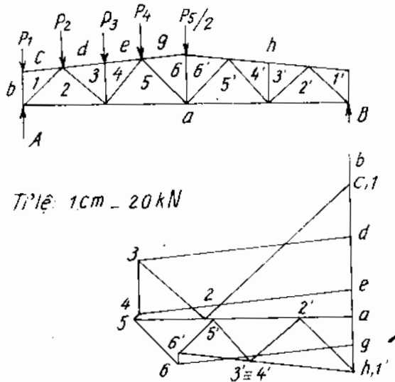
Hình 4.7. Đồ giải Crémone của hoạt tải ở nửa trái dầm
