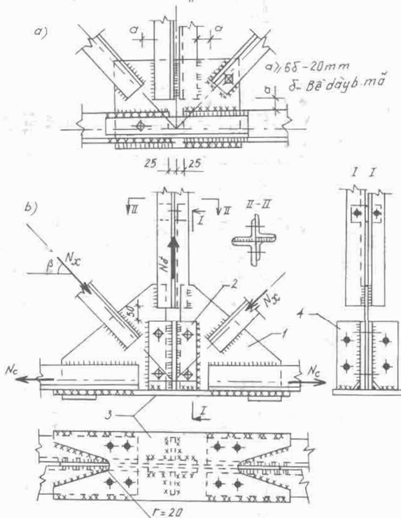
Hình 4.19. Nút giữa dưới
