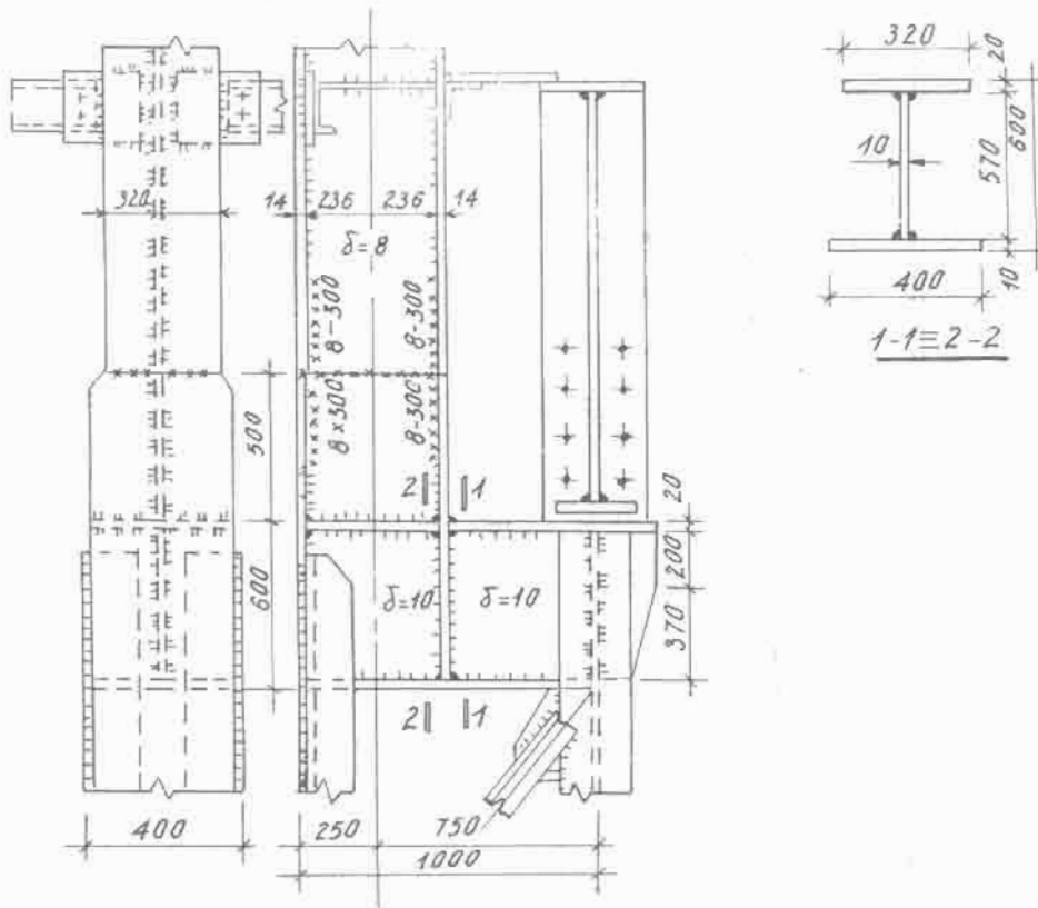
Hình 3.14. Nối cột trên với cột dưới rộng. Liên kết dầm cầu chày và cánh dầm hãm với cột
