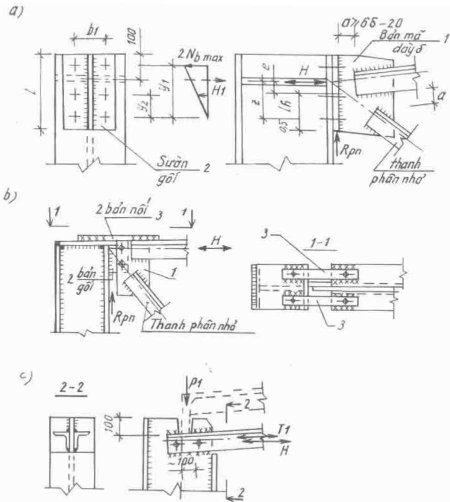
Hình 4.22. Nút trên đầu dầm liên kết cứng với cột
