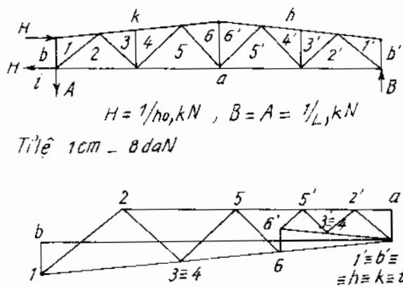
Hình 4.8. Đồ giải Crémone với M = +1 ở đầu trái
