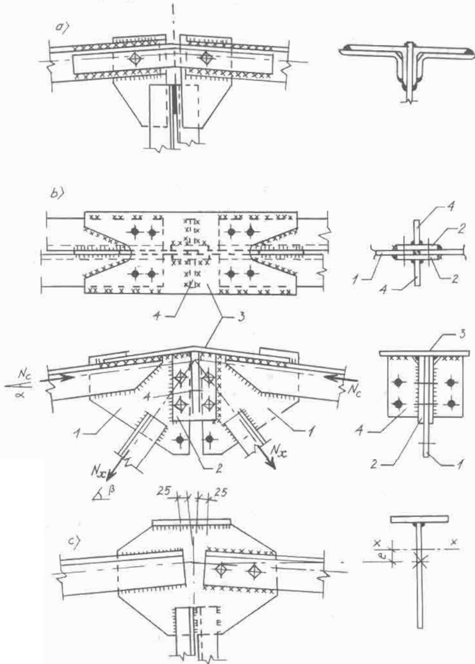
Hình 4.18. Nút dính dãn
