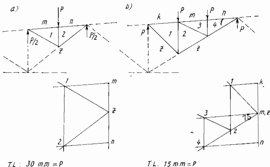
Hình 4.9. Đồ giải Crémone của dầm phân nhỏ
