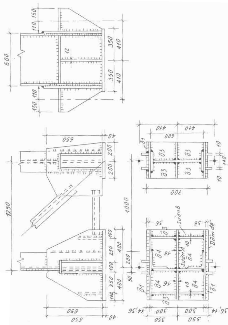
Hình 3.18. Chân cột rộng ở vị trí 3.5
