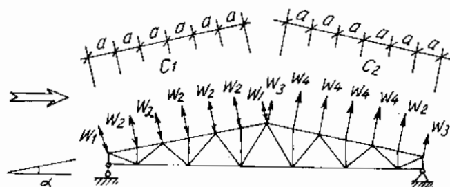
Hình 4.4 Sơ đồ tải trọng gió trên vì kèo
