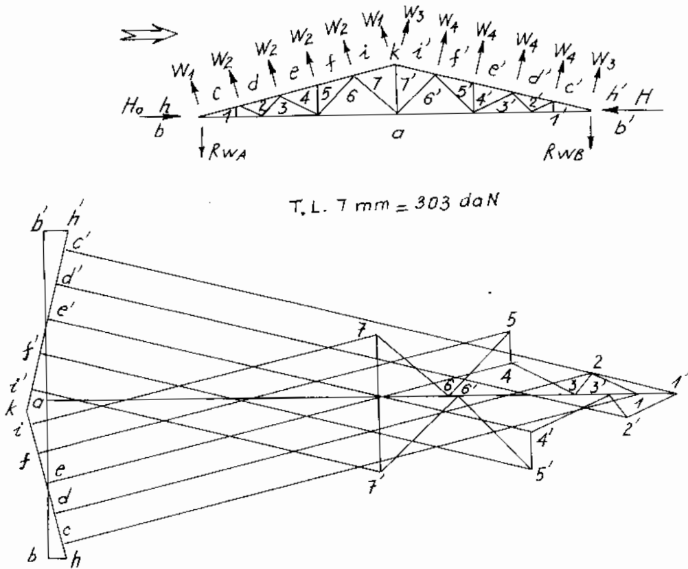
Hình 4.12. Đồ giải Crêmona với tải trọng gió của dàn vì kèo cho ví dụ 4.1
