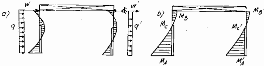
Hình 2.9. Tính với tải trọng gió
