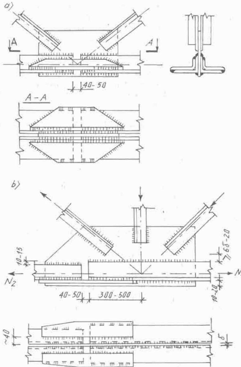
Hình 4.17. Nút trung gian có nối thanh cánh:
