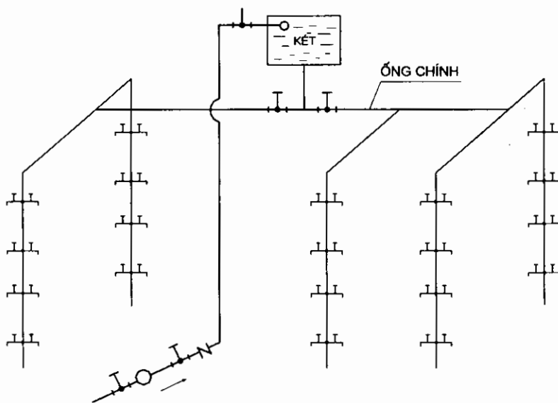
Hình 2.13: Sơ đồ có két nước trên mái
