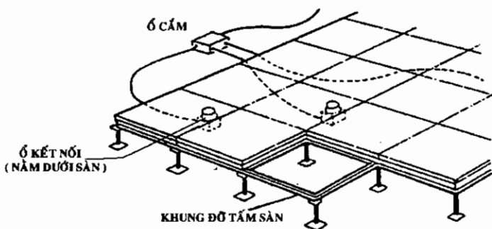
Hình 1.4: Sàn kỹ thuật rỗng kiểu khung giá đỡ định hình
