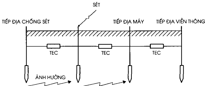
Hình 3.23: Van TEC
