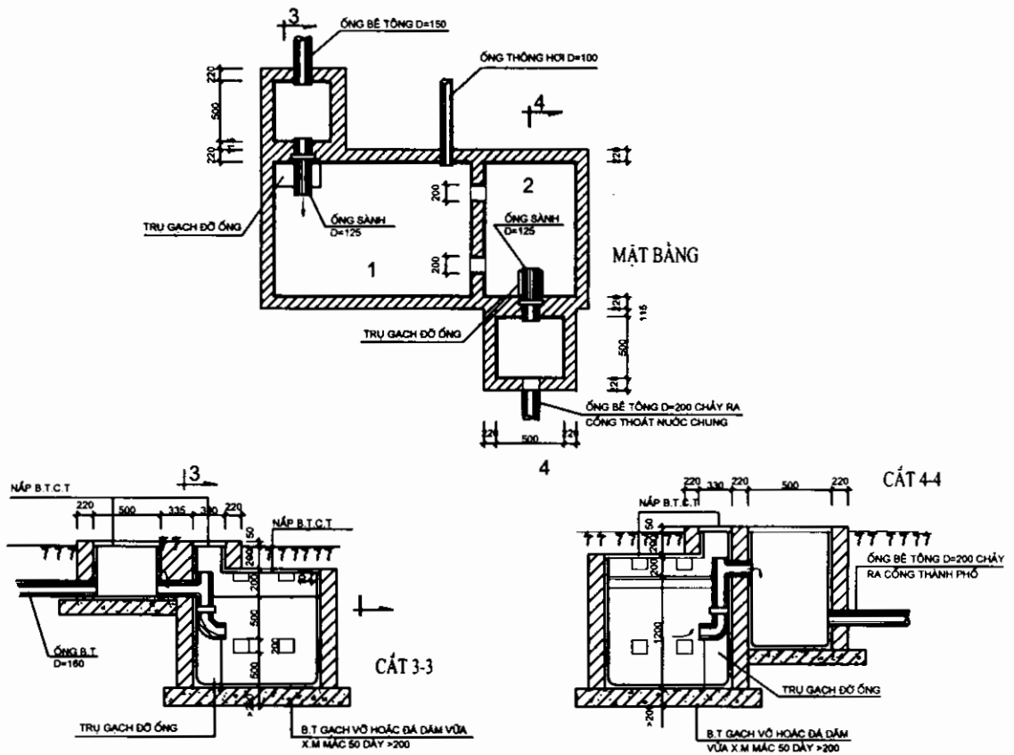
Hình 2.23: Bể tự hoại kiểu lửng
