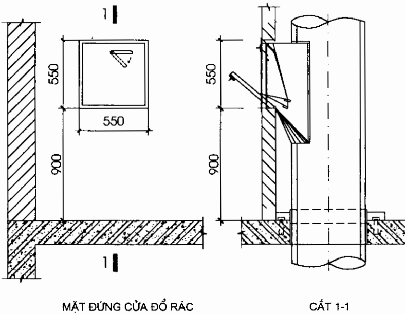
Hình 8.6. Chi tiết cửa đổ rác bằng sắt không gỉ.
