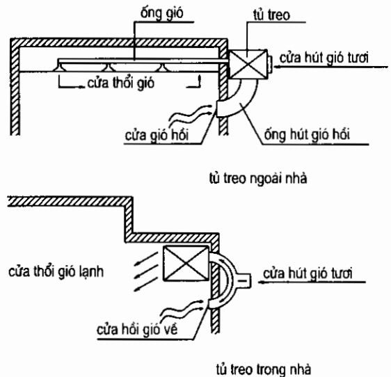
Hình 5.17: Giàn lạnh tủ kiểu treo
