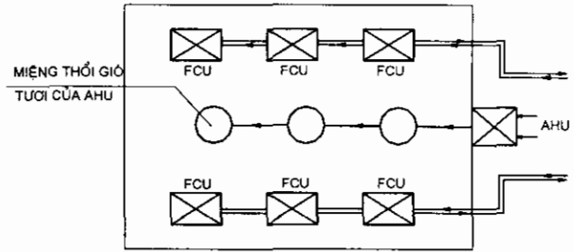
Hình 5.28: Bố trí xen kẽ AHU và FCU
