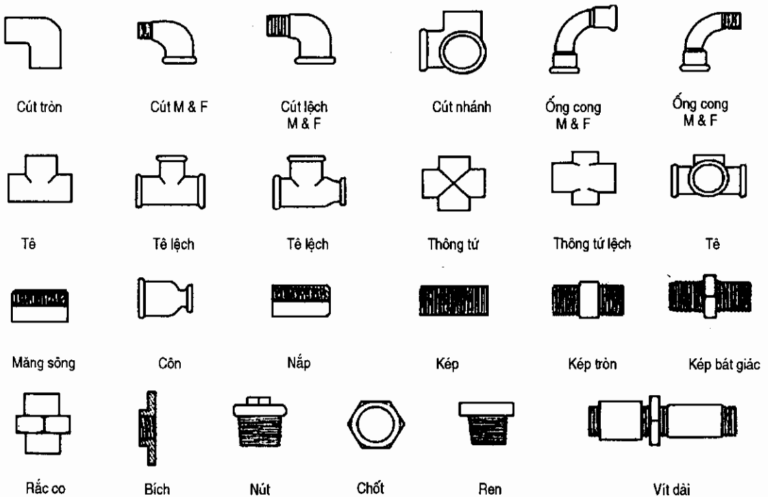
Hình 2.3: Phụ tùng nối ống kẽm
