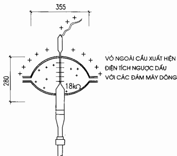
Hình 3.18: Kim thu sét Dynasphee – ESE
