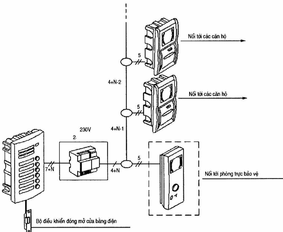
Sơ đồ nối của hệ thống video door entry - nhiều máy
