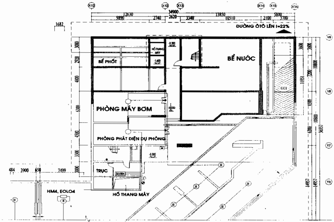
Hình 1.12: Mặt bằng phòng kỹ thuật máy bơm, máy phát điện trong một công trình
