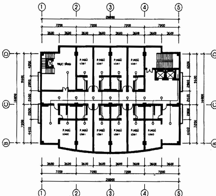
MẶT BẰNG TẦNG KS ĐIỂN HÌNH
