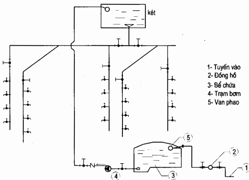
Hình 2.14: Sơ đồ có bể chứa, trạm bơm và két nước trên mái
