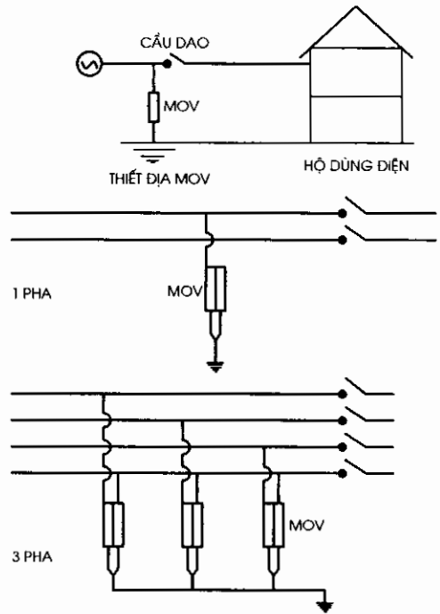
Hình 3.21: Bộ phận cắt sét MOV
