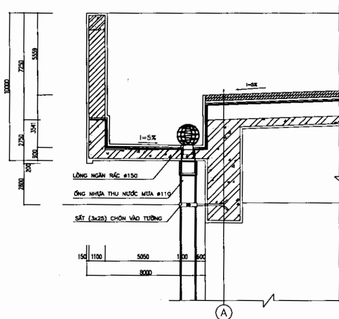
Hình 2.24: Liên kết phễu thu với kết cấu mái
