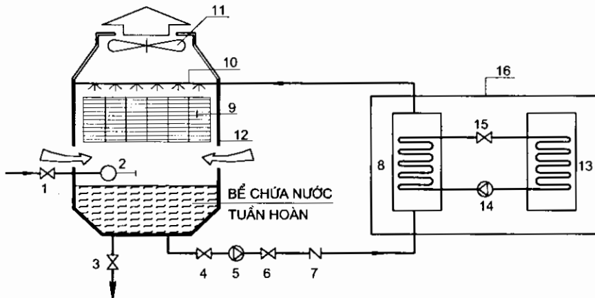
Hình 5.18: Tháp giải nhiệt
