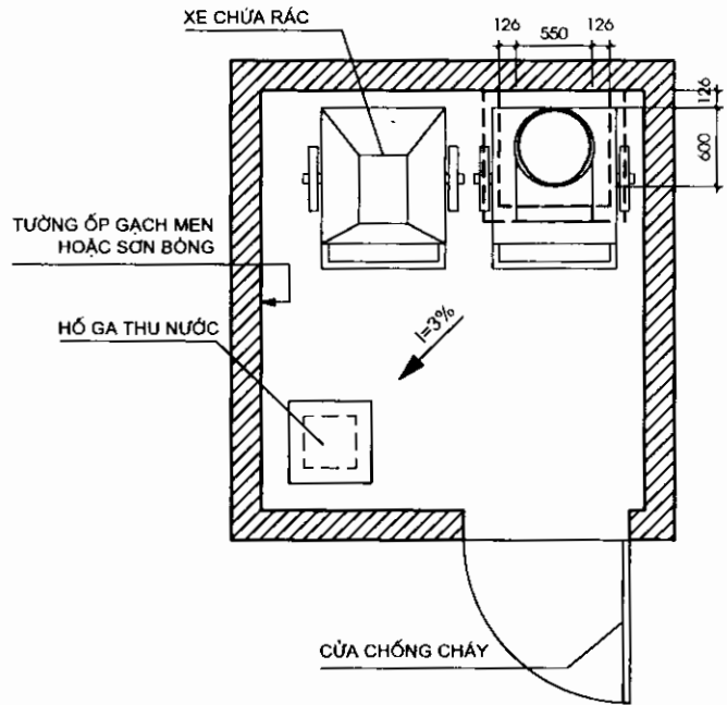
Hình 8.12: Ví dụ mặt bằng một phòng thu rác với cách bố trí xe chứa rác, ga thu nước bản, vật liệu sử dụng...
