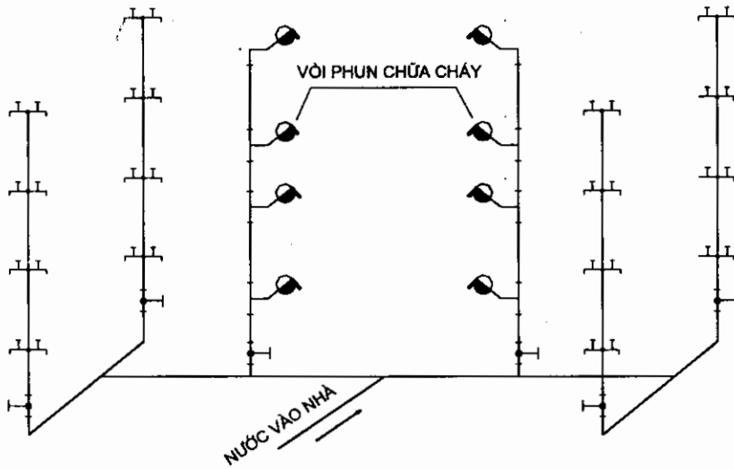
Hình 2.16: Sơ đồ hệ thống cứu hoả bán cố định (cứu hoả vách tường) kết hợp với hệ thống cấp nước sinh hoạt
