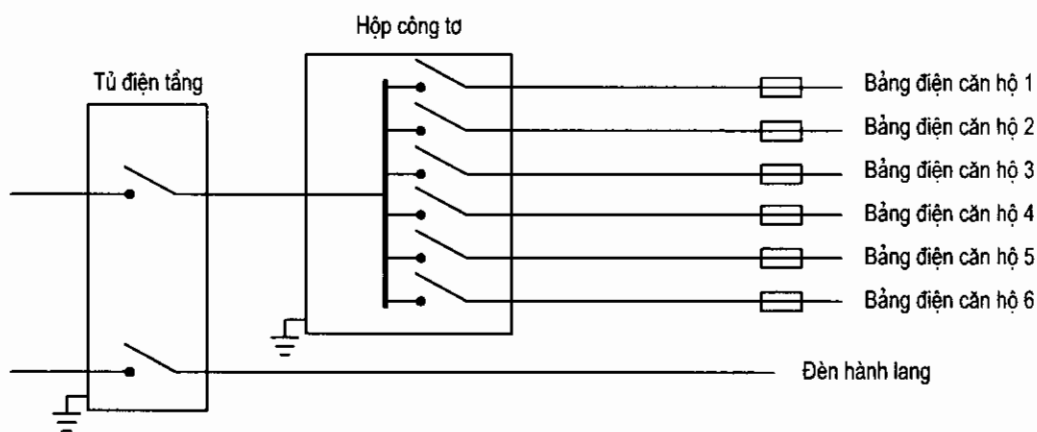
Hình 3.4a: Sơ đồ phân phối điện từ tủ điện tầng đến tủ điện căn hộ
