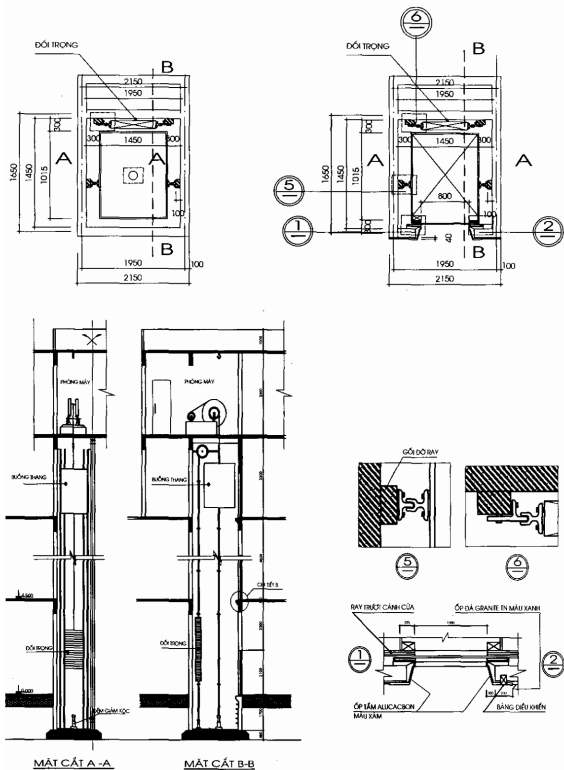
Hình 6.7: Thang máy có đối trọng (tham khảo)
