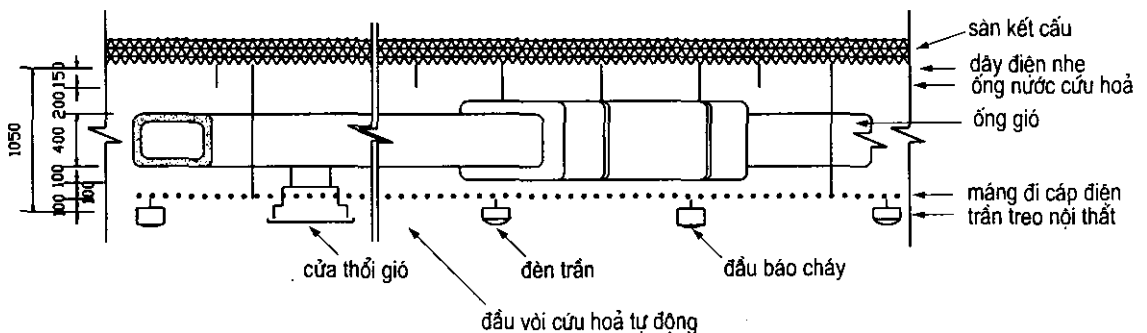
Hình 9.3. Sơ đồ mặt cắt thể hiện các lớp đường ống thiết bị trong trần kỹ thuật
