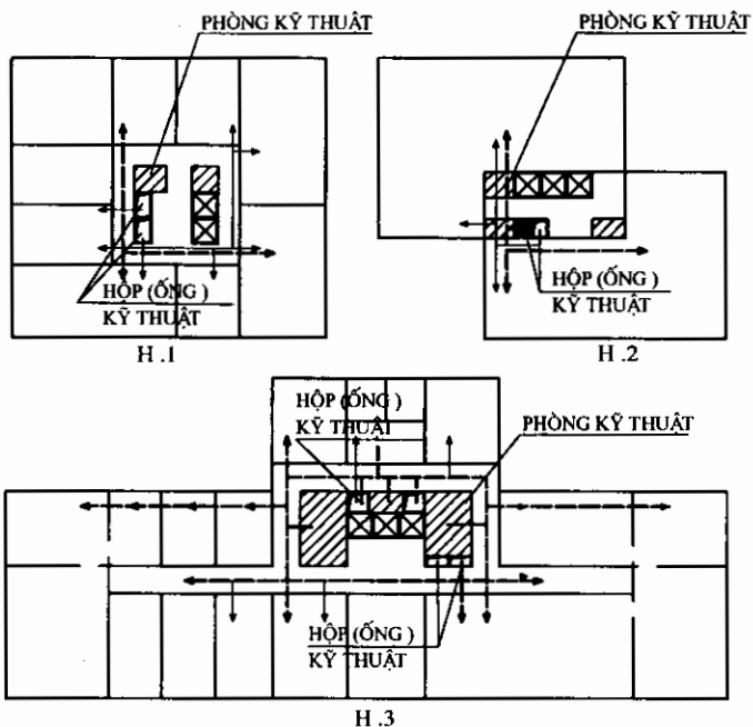
H.1,2,3 : HỘP KỸ THUẬT ĐƯỢC BỐ TRÍ Ở TRUNG TÂM MẶT BẰNG (LỖ)
