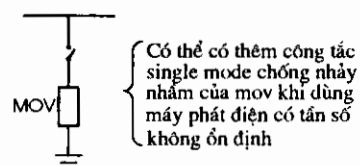
Hình 3.22: Thiết bị cắt lọc sét kiểu SRF
