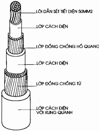
Hình 3.19: Cáp Triax
