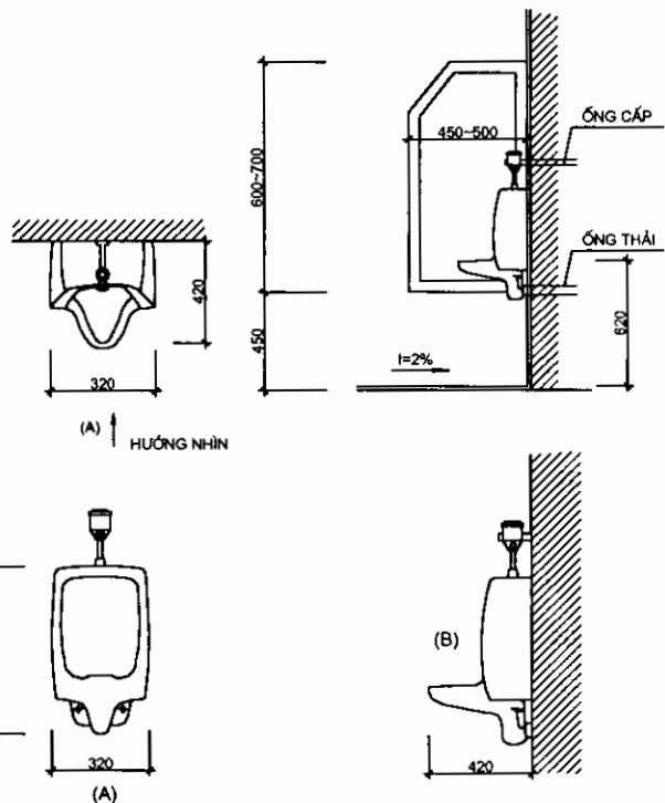
Hình 2.8: Âu tiểu nam
