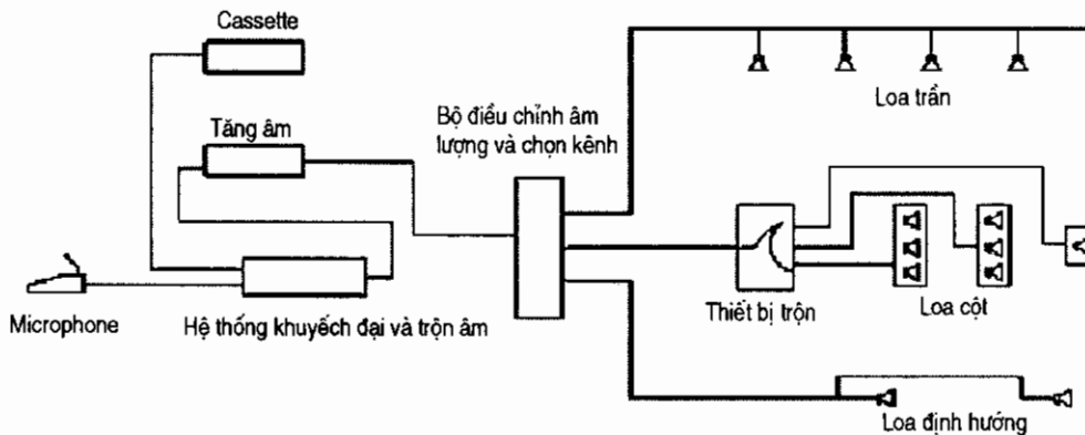
Hình 7.10. Sơ đồ hệ thống âm thanh thông báo công cộng
