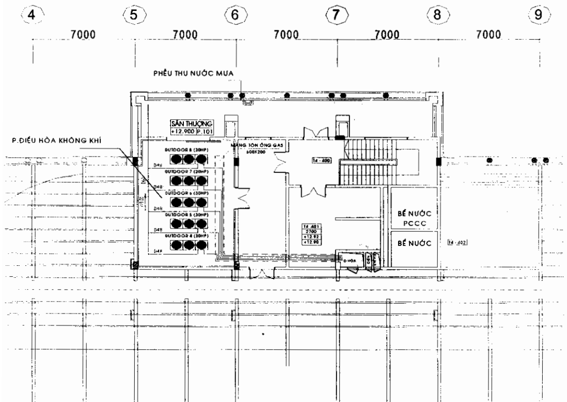
Hình 1.14: Mặt bằng phòng kỹ thuật máy điều hoà trung tâm trong một công trình
