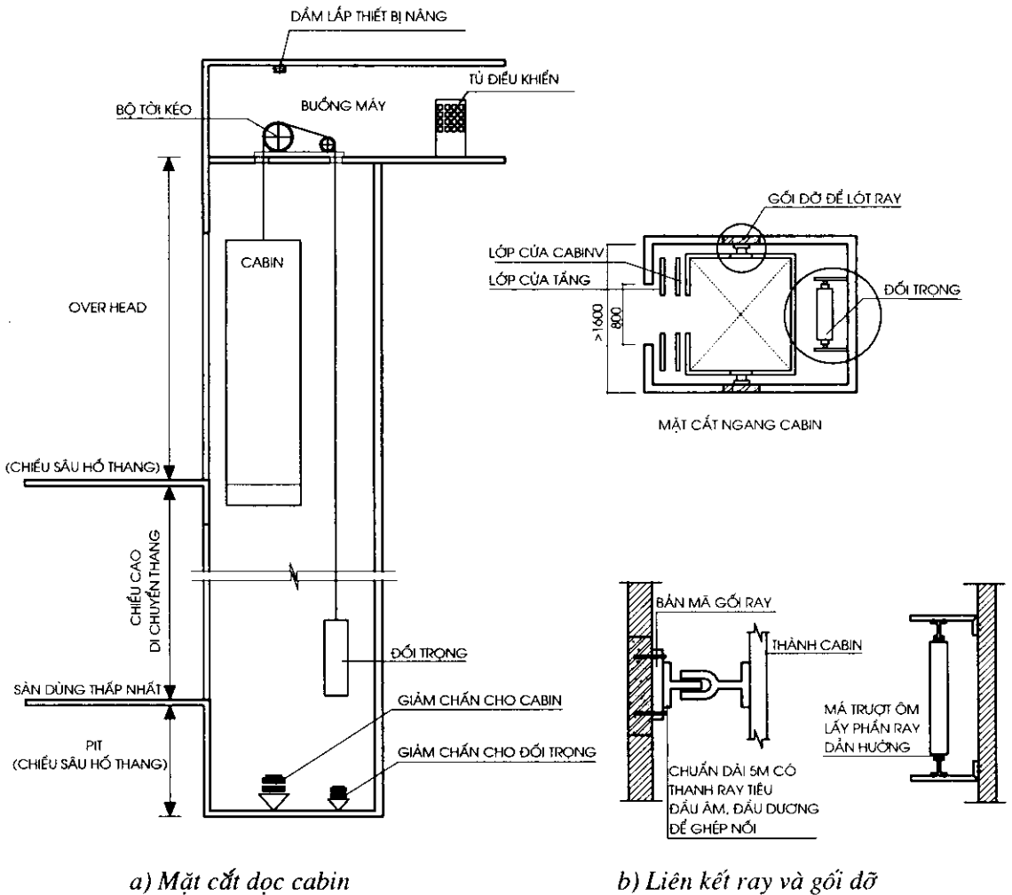
Hình 6.3: Cấu tạo Carbin với giăng thang và đối trọng
