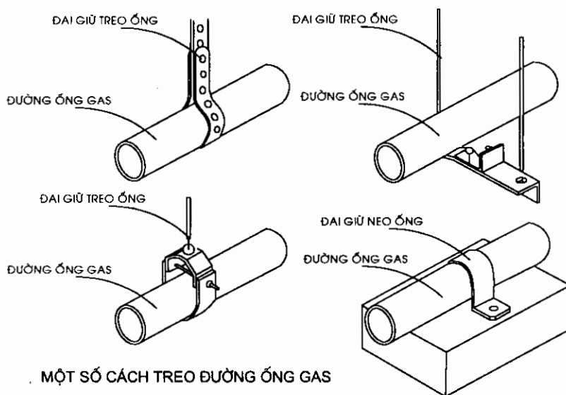
Hình 8.3. Chi tiết treo ống
