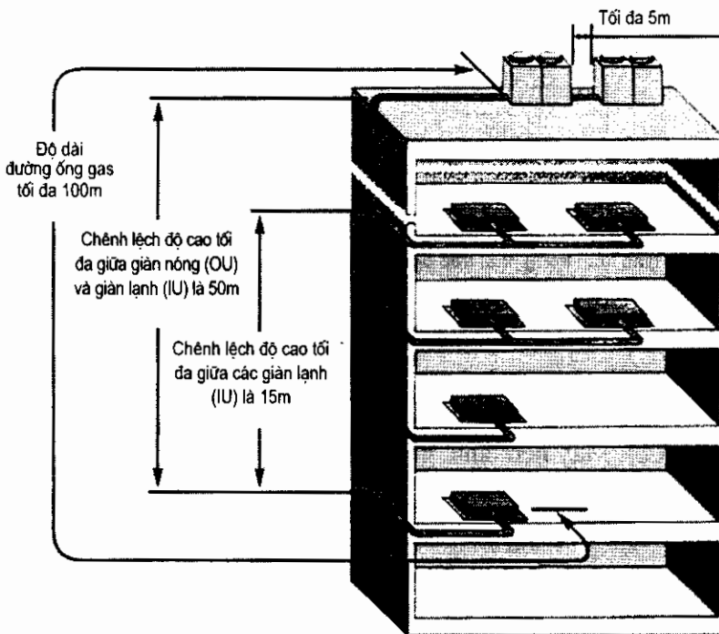
Hình 5.24: Lắp đặt hệ thống máy điều hoà không khí trung tâm VRV
