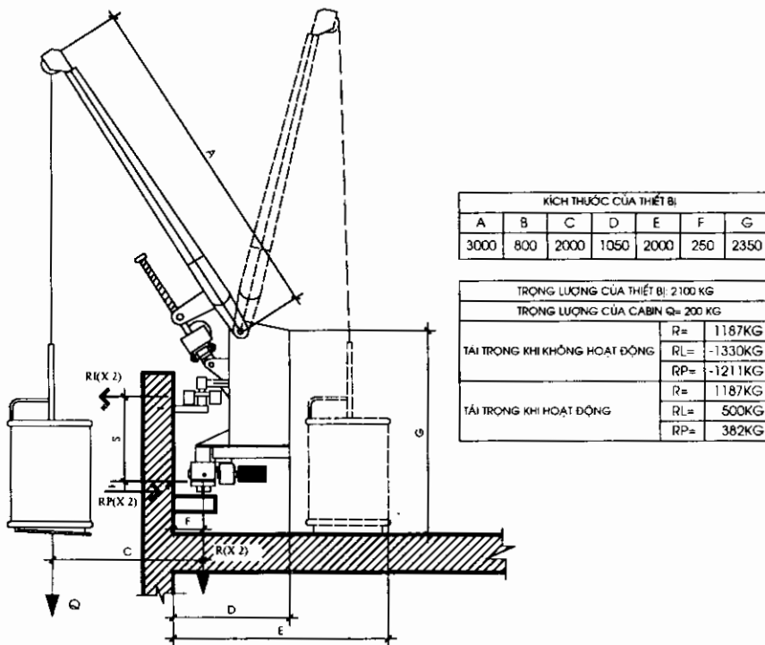
Hình 8.14. Cần cấu mini để thả cabin
