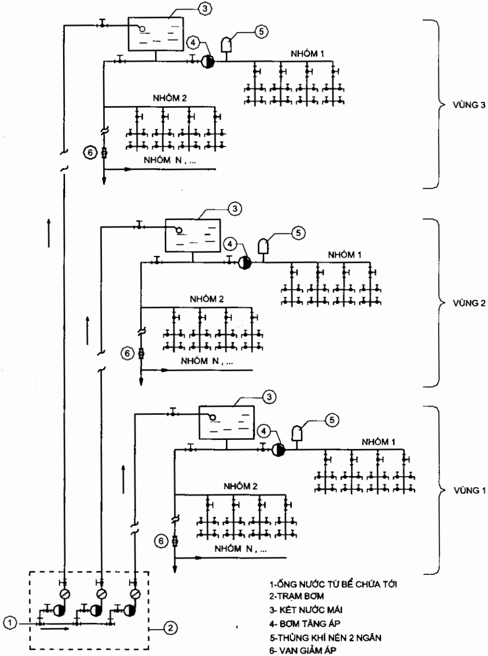
Hình 2.15: Sơ đồ cấp nước phân vùng
