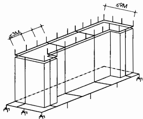
Hình 3.13: Chống sét kiểu lồng Faraday
