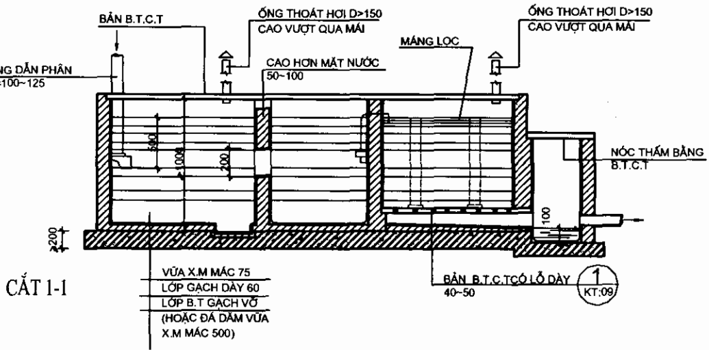
Hình 2.22: Bể tự hoại loại có ngăn lọc
