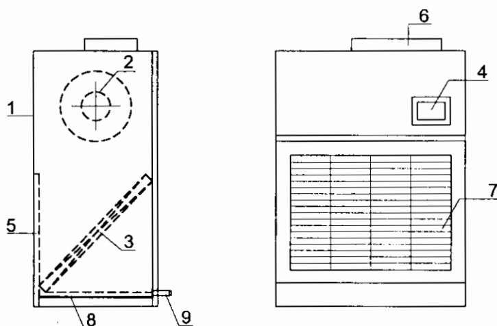
Hình 5.15: Điều hoà không khí dạng tủ
