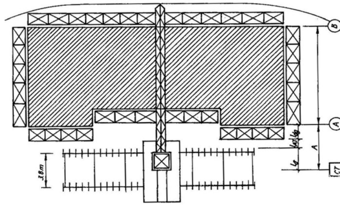
Hình 6-1b. Mặt bằng bố trí cần trục chạy trên ray có đối trọng ở dưới.
