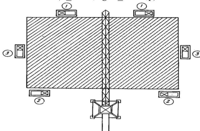
Hình 6-6. Bố trí thang tải khi có cần trục tháp đứng cố định.
