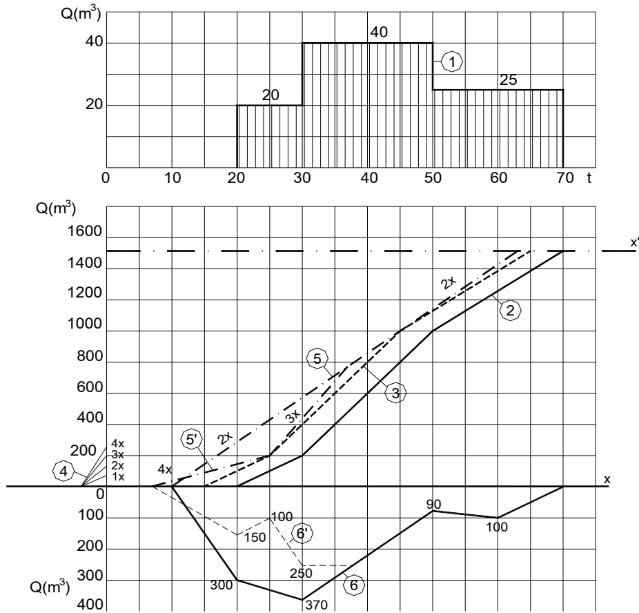
Hình 4-3. Biểu đồ vật tư.
