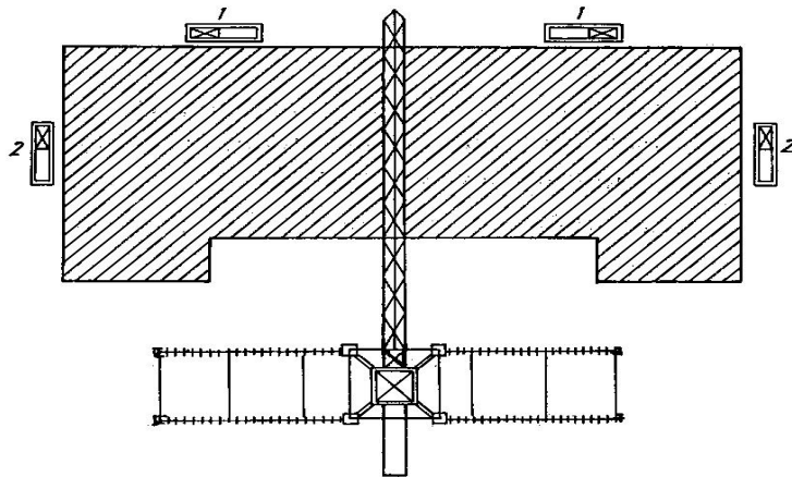
Hình 6-5. Bố trí thang tải khi có cần trục chạy trên ray (1_MB rộng, 2_MB hẹp).
