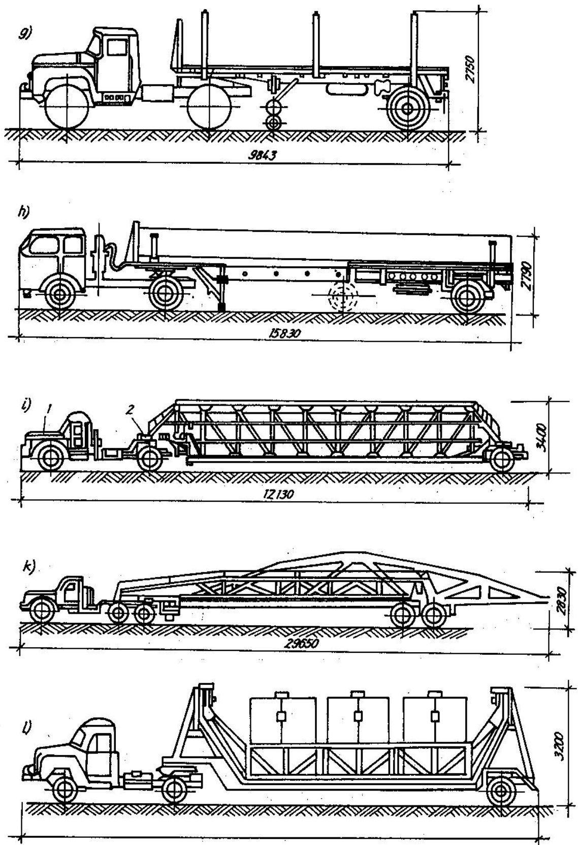
Hình 7-1. Một số loại xe vận chuyển trong xây dựng. a) Xe ô tô có thùng; b) Xe ô tô có bệ; c) Xe ô tô có thùng tự đổ; d) Xe chở vữa; e) Xe chở bê tông; g) Xe chở tấm tường, tấm sàn; h) Xe chở dầm; i) Xe chở panen; k) Xe chở dầm; l) Xe chở thùng.
