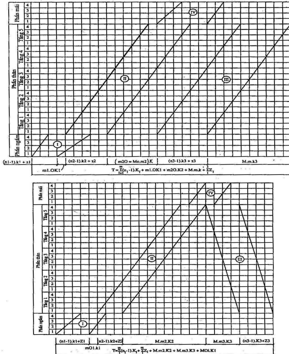
Hình 4-2. Công tác hoàn thiện công trình nhiều tầng.
