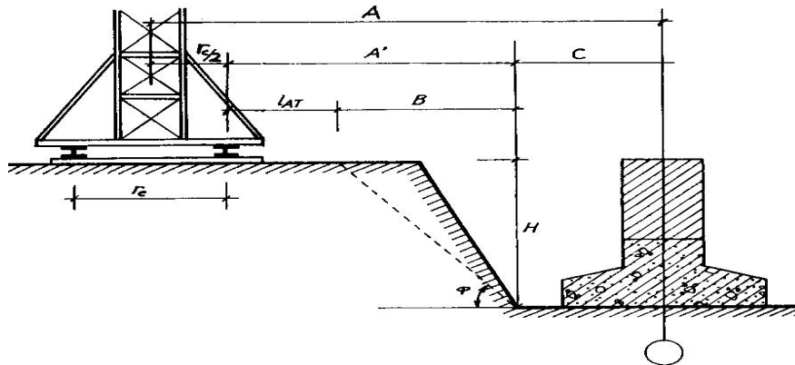
Hình 6-4. Vị trí cần trục tháp loại chạy trên ray khi thi công phân ngầm.
