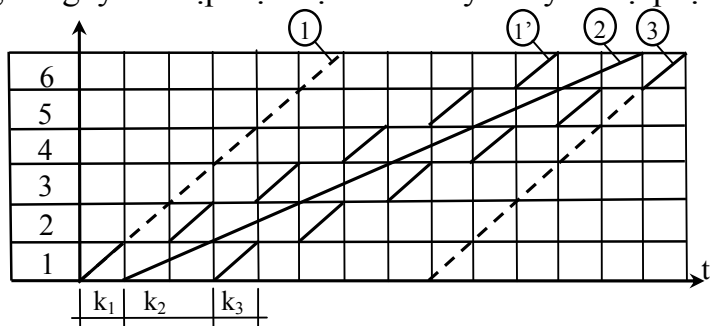
Cân bằng dây chuyền bộ phận theo nhịp độ chậm
