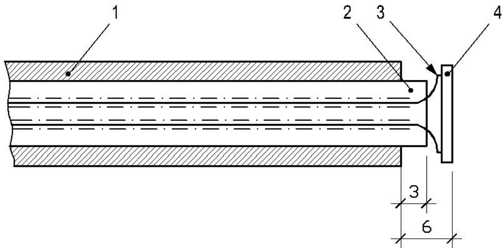
Hình 2- cặp nhiệt ngẫu và đệm cách ly của bề mặt không tiếp xúc với lửa
