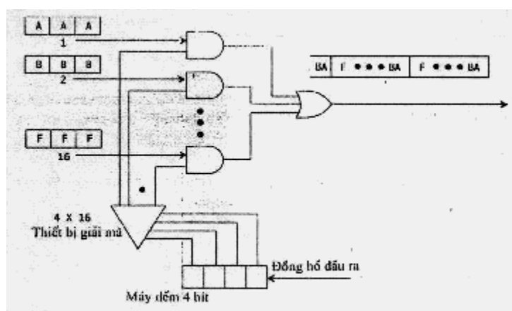
Hình 3.5. Bộ ghép kênh TDM 16:1
