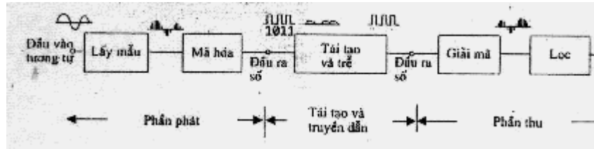
Hình 3.8. Cấu hình cơ bản phương pháp thông tin PCM
