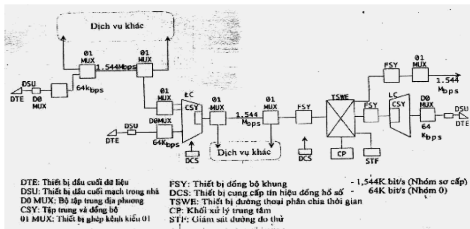
Hình 2.20. Phương pháp rơ-le của mạng chuyển mạch tuyến
