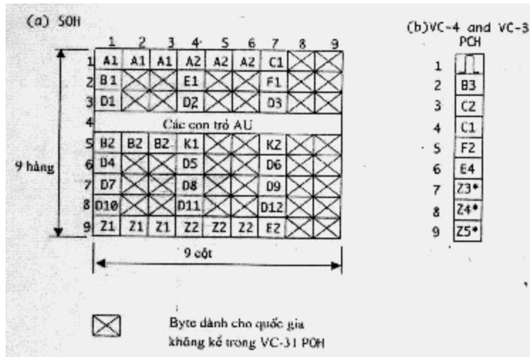
Hình 3.34. Phần tử bố xung của khung STM.1.
