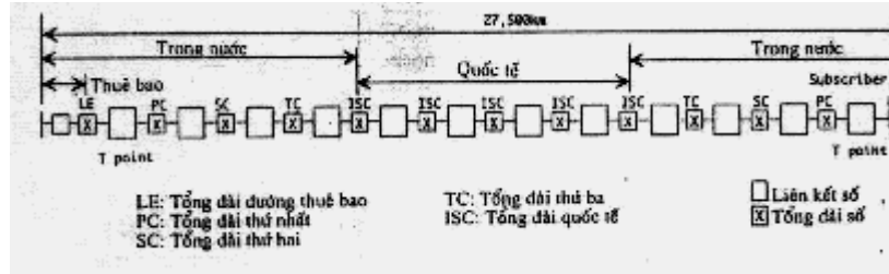
Hình 3.3. HRX tiêu chuẩn quốc tế (cấp dài nhất)
