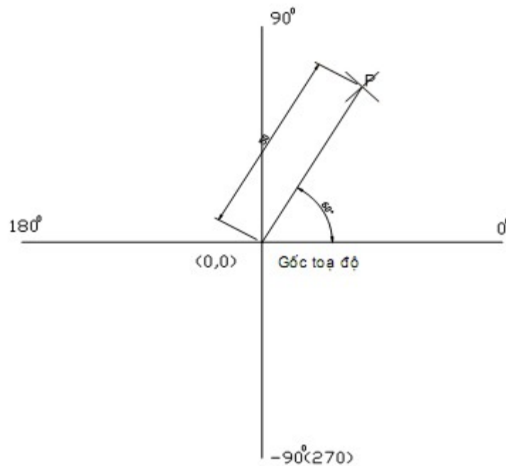
Hệ tọa độ cực
