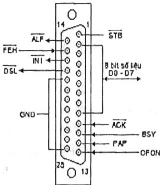
Đầu nối D - 25 cho cổng LPT
