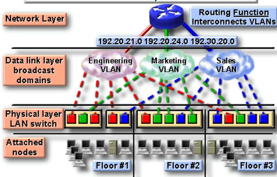
Hình 6.5 – Cài đặt VLAN dựa trên cổng
