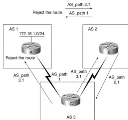
Hình 5.17 – Sử dụng thuộc tính AS_path trong BGP
