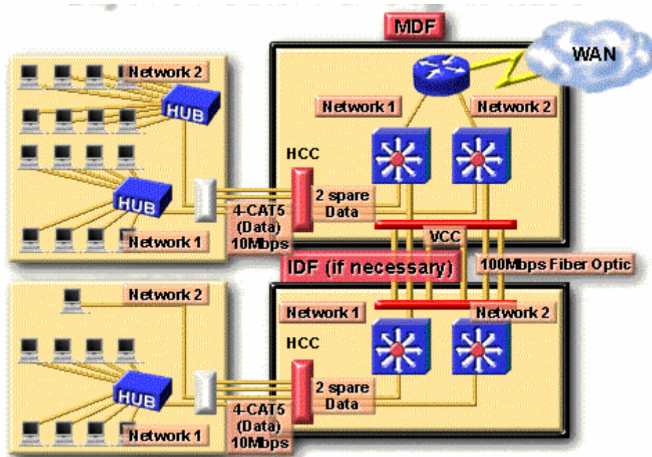
Hình 7.15 – Sử dụng router để phân chia vùng đưng độ trong mạng
