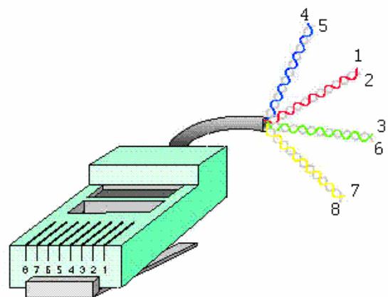
Hình 2.7 – Sử dụng đầu nối UTP với dây cáp xoắn đôi
