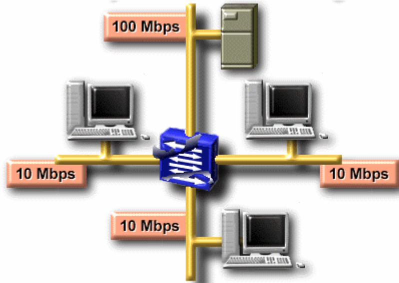
Hình 4.8 – Asymmetric switch
