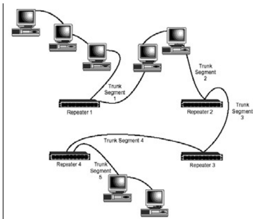
Hình 2.7 – Quy tắc 5-4-3.
