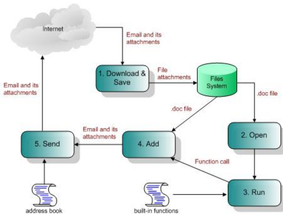
Các bước hoạt động của virus Melissa
