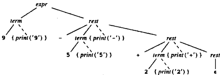
Hình 2.21. Dịch 9-5+2 thành 95-2+ .
