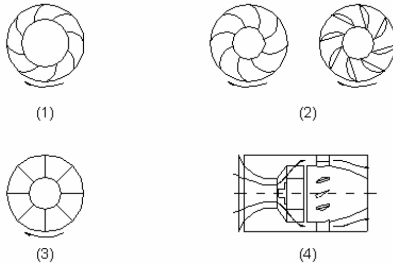
Hình 6-26 : Các loại quạt ly tâm
