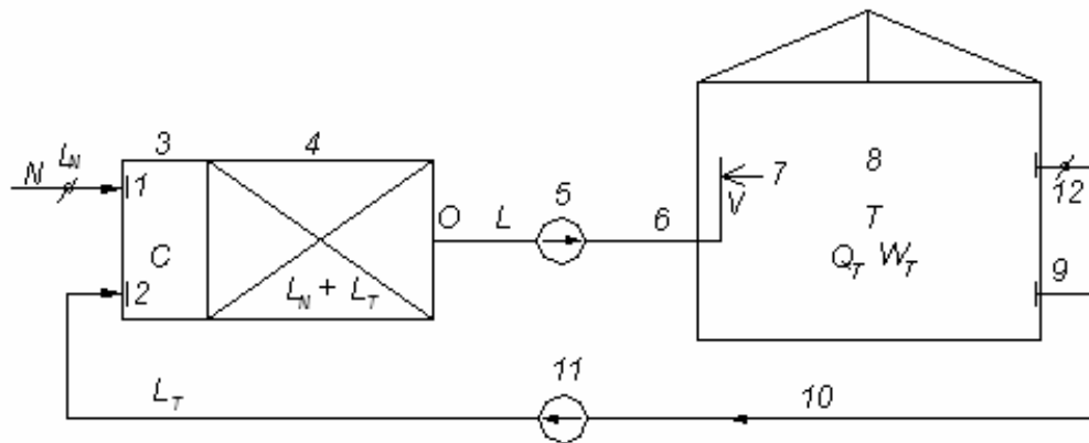
Hình 4.13: Sơ đồ tuần hoàn 1 cấp mùa đông
