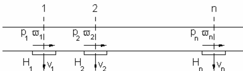
Hình 6.2 : Phân bố cột áp tĩnh dọc theo kênh gió
