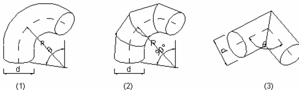
Hình 6-5: Cút tiết diện tròn
