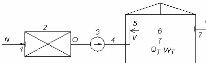
Hình 4.11: Sơ đồ thẳng mùa đông
