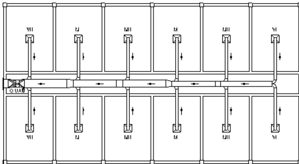
Hình 8-4 : Sơ đồ bố trí quạt thông gió
