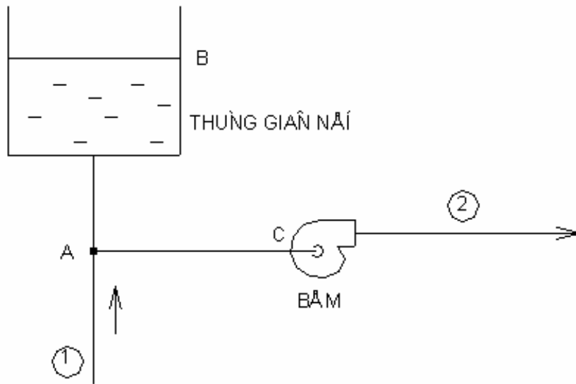
Hình 7-5 : Lắp đặt thùng giãn nở
