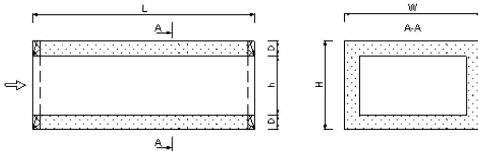
Hình 9-2 : Cấu tạo hộp tiêu âm
