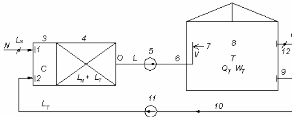
Hình 4.3 Sơ đồ tuần hoàn 1 cấp
