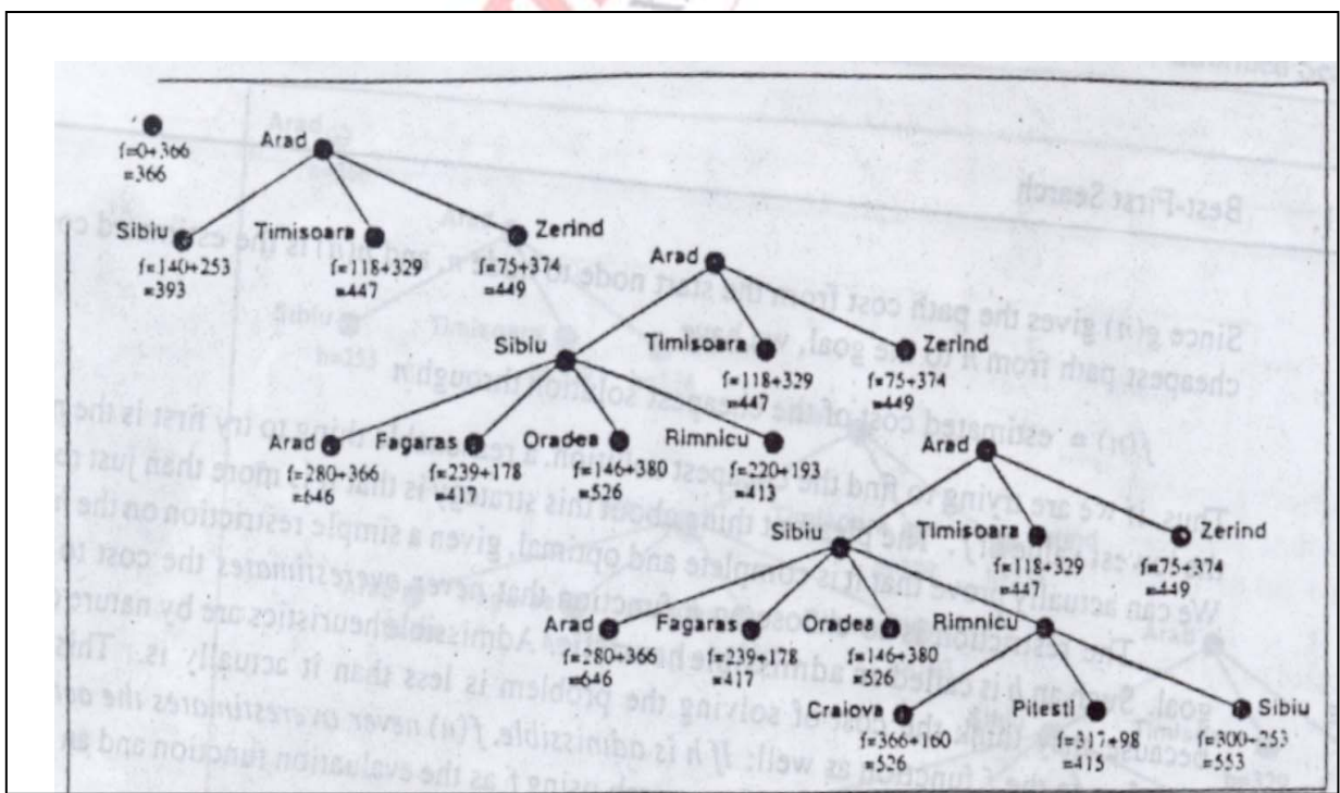
Hình 2.8 Các giai đoạn của phép tìm kiếm A để đi đến Bucharest. Các nút được gán nhãn với f = g + h . Các giá trị h là các khoảng cách đường thẳng tới Bucharest lấy từ giả thiết
