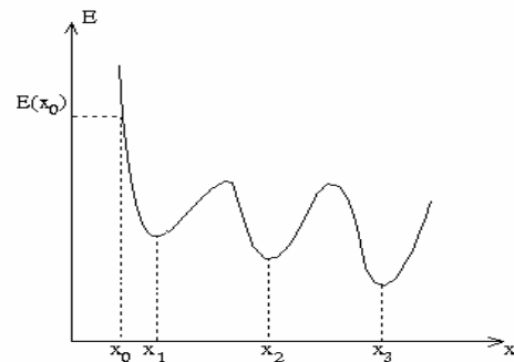
Hình 5.6: Năng lượng mạng E(x)
