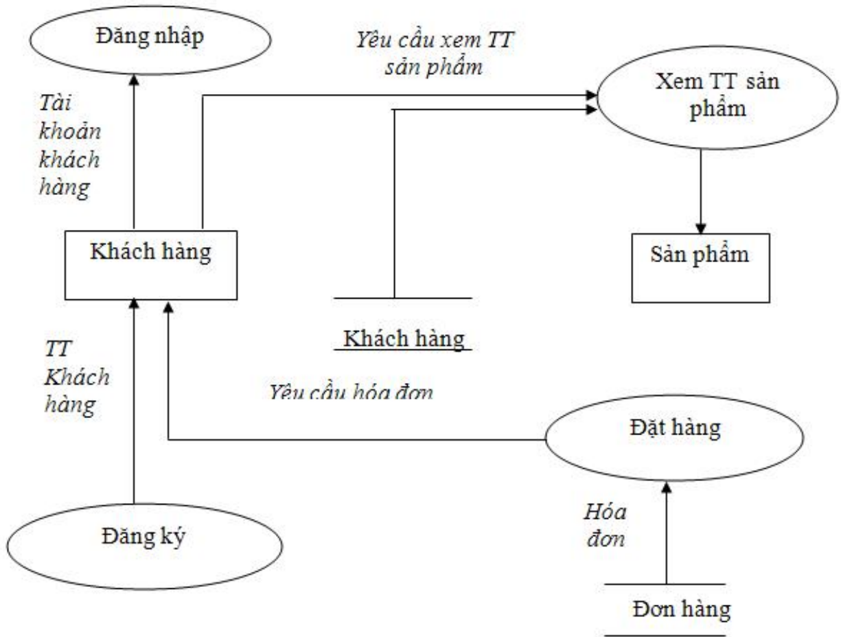
Biểu đồ luồng dữ liệu mức 1 của chức năng giao dịch
