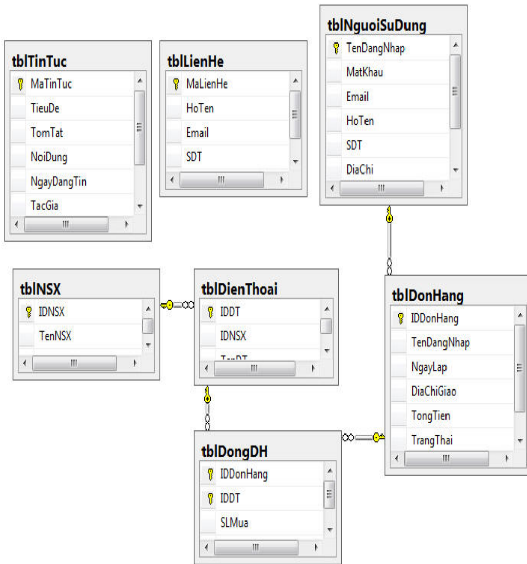
Sơ đồ quan hệ cơ sở dữ liệu
