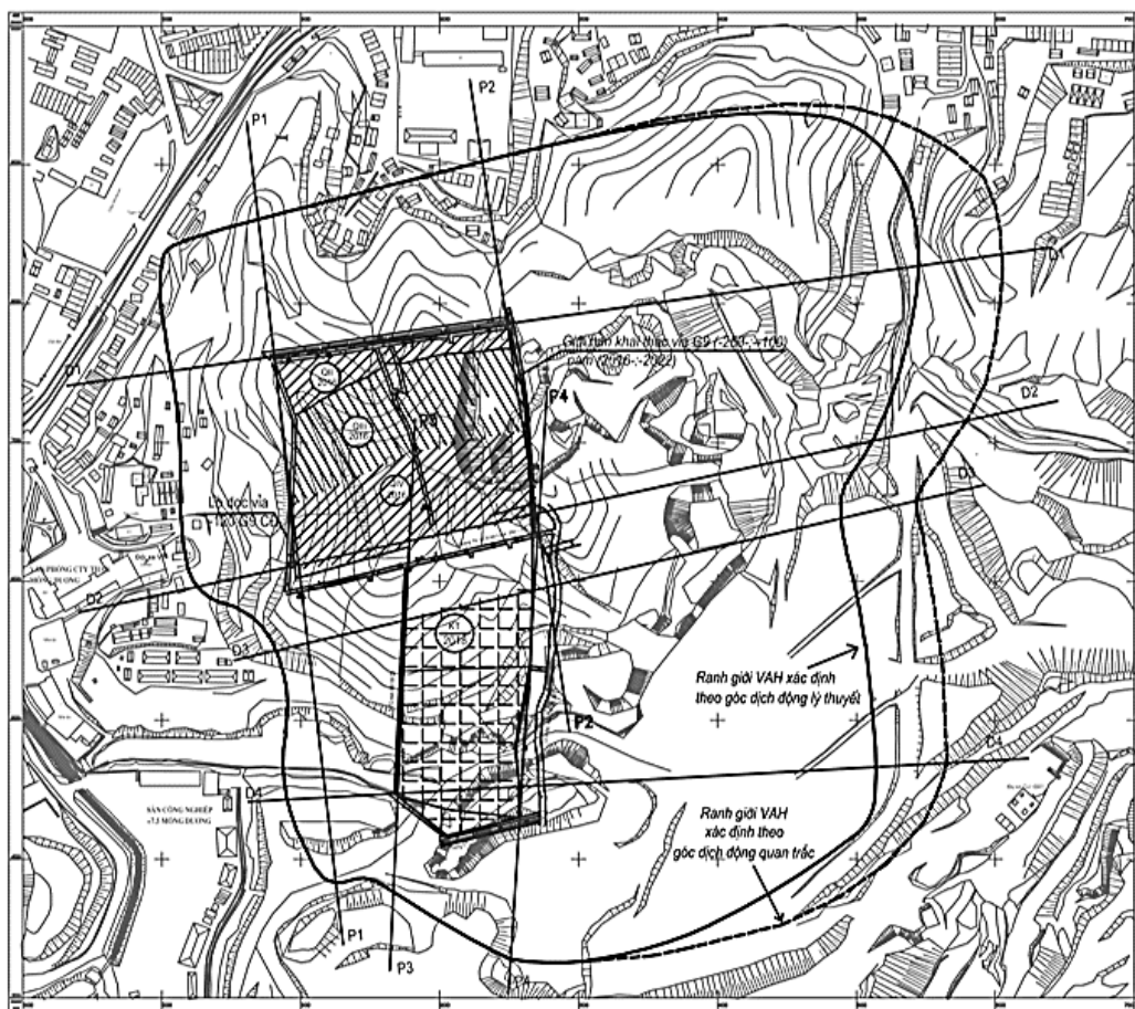
Hình 7. Ranh giới dịch động do khai thác vỉa G9CĐ mở Mông Dương.
