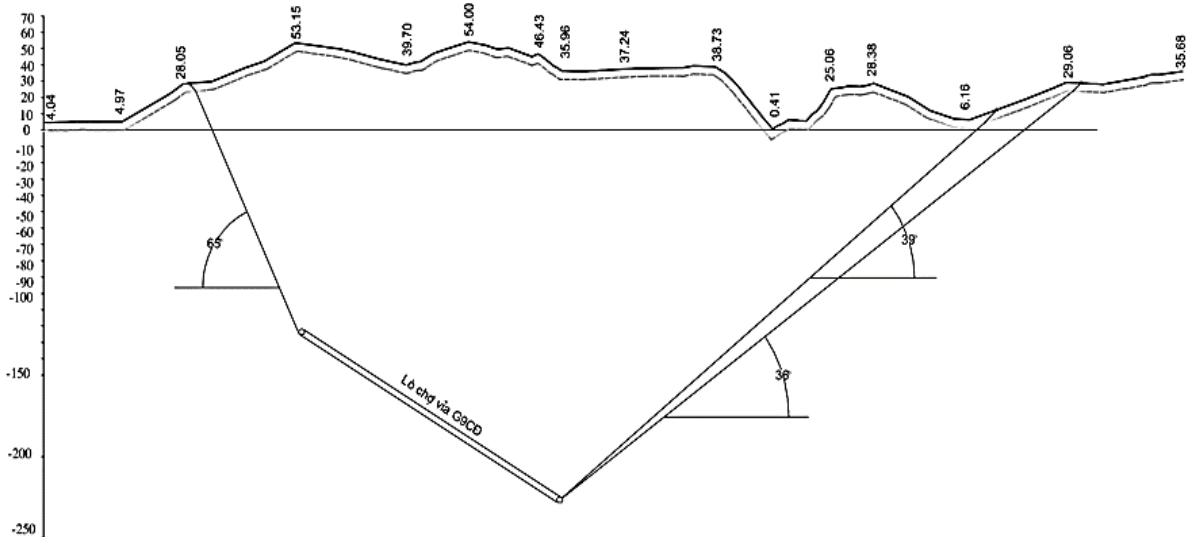
Hình 5. Mặt cắt theo dốc D1-D1.
