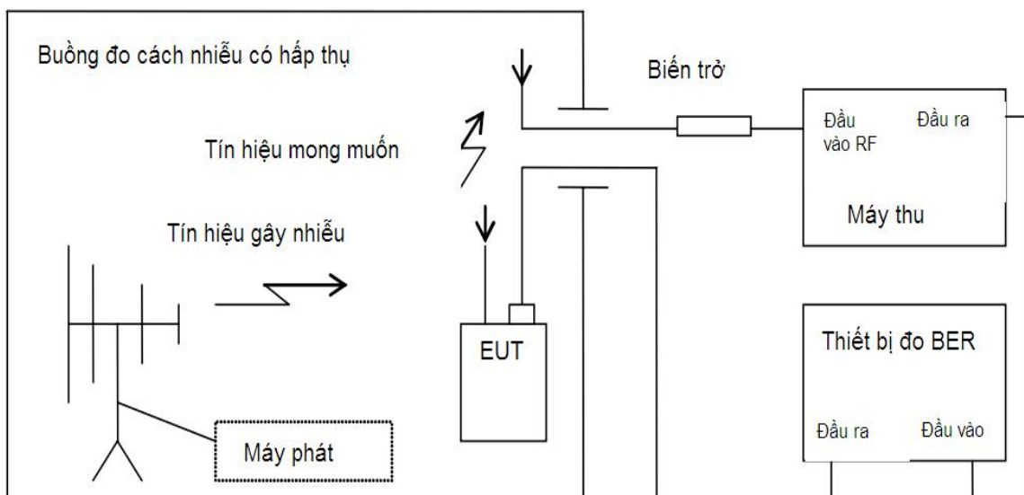
Hình 2- Cấu hình đo ăng ten liền; hoạt động của máy phát - đầu vào dòng điện
