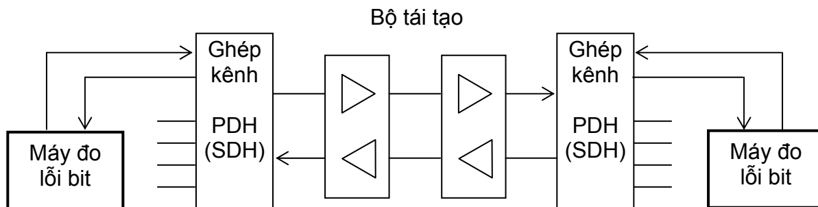
Hình 7 - Đo lỗi khối đầu cuối đến đầu cuối
