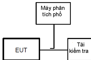
Hình 10 - Sơ đồ đo mật độ công suất của đầu ra phát
