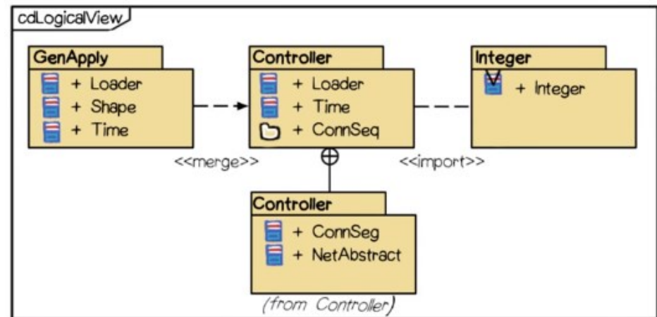
UML 2.0
