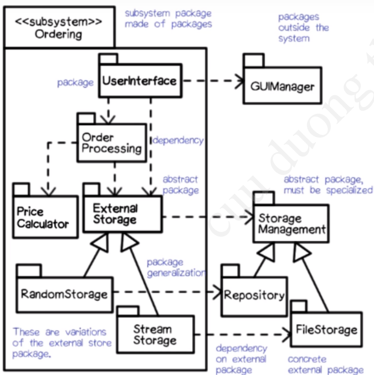
UML 1.5
