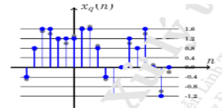
(e) Tín hiệu đã lượng tử hóa
